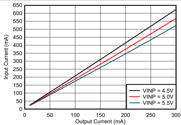
图 6-15. 输入电流 ( I_{VINP} ) 与负载电流 ( I_{VCC} ) 间的关系: V_{CC} = 5.0\text{V} , T_A = 25^\circ\text{C} , C_{OUT2} = 22\text{ }\mu\text{F}
