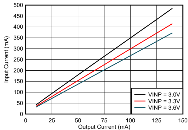
图 6-17. 输入电流 ( I_{VINP} ) 与负载电流 ( I_{VCC} ) 间的关系: V_{CC} = 5.0\text{V} , T_A = 25^\circ\text{C} , C_{OUT2} = 22\text{ }\mu\text{F}
