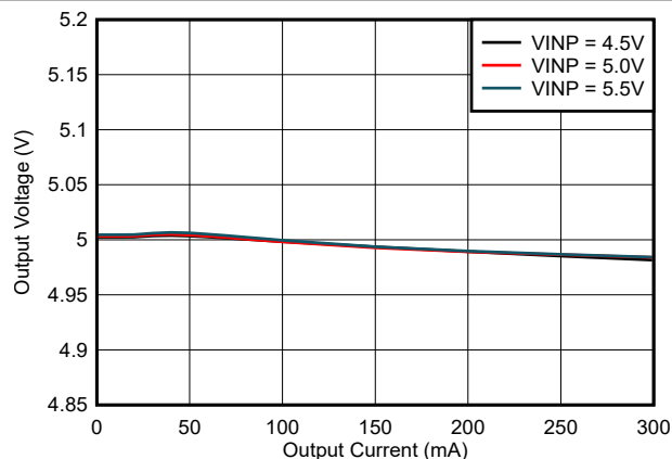
图 6-19. 输出电压调节 ( V_{VCC} ) 与负载电流 ( I_{VCC} ) 间的关系: V_{CC} = 5.0V , T_A = 25^\circ C , C_{OUT2} = 22 \mu F
