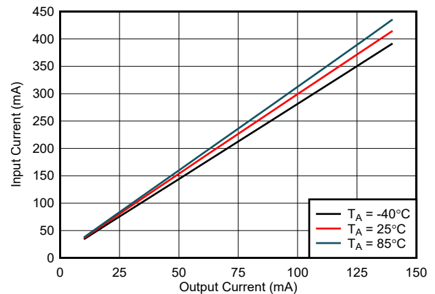
图 6-18. 输入电流 ( I_{VINP} ) 与负载电流 ( I_{VCC} ) 间的关系: V_{CC} = 5.0\text{V} , V_{INP} = 3.3\text{V} , C_{OUT2} = 22\text{ }\mu\text{F}
