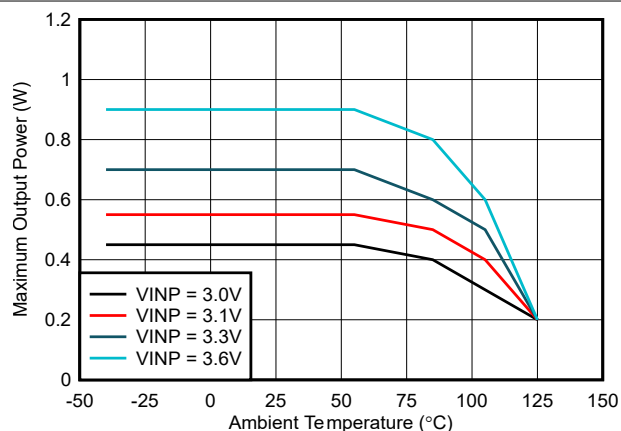
图 6-4. 最大输出功率与环境温度间的关系：VCC = 5.5V，COUT2 = 22 μF
