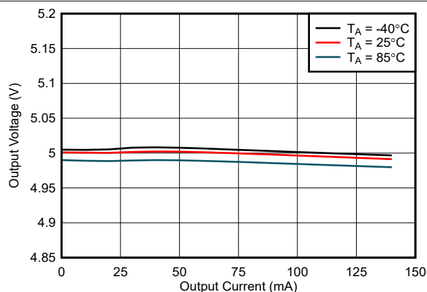
图 6-23. 输出电压调节 ( V_{VCC} ) 与负载电流 ( I_{VCC} ) 间的关系: V_{CC} = 5.0V , V_{INP} = 3.3V , C_{OUT2} = 22 \mu F
