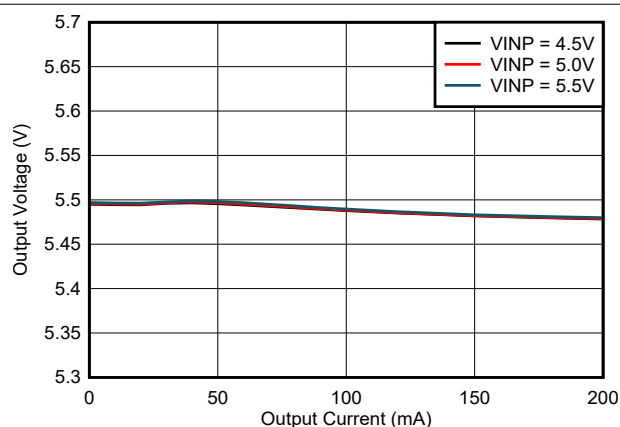
图 6-21. 输出电压调节 ( V_{VCC} ) 与负载电流 ( I_{VCC} ) 间的关系: V_{CC} = 5.5V , T_A = 25^\circ C , C_{OUT2} = 22 \mu F
