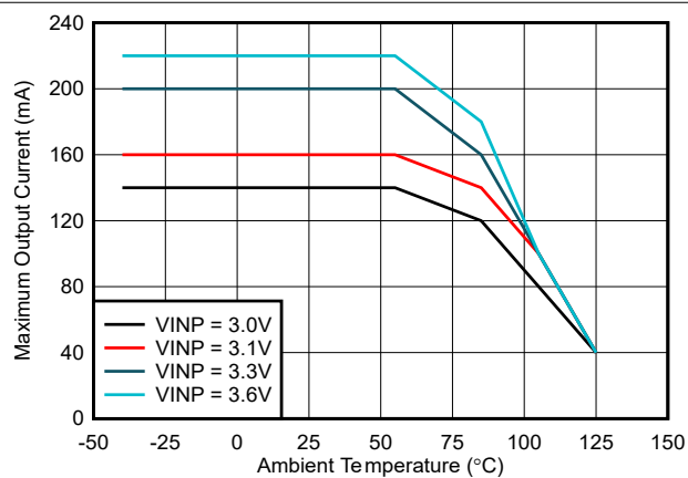
图 6-6. 最大输出电流与环境温度间的关系：VCC = 5.0V，COUT2 = 22 μF
