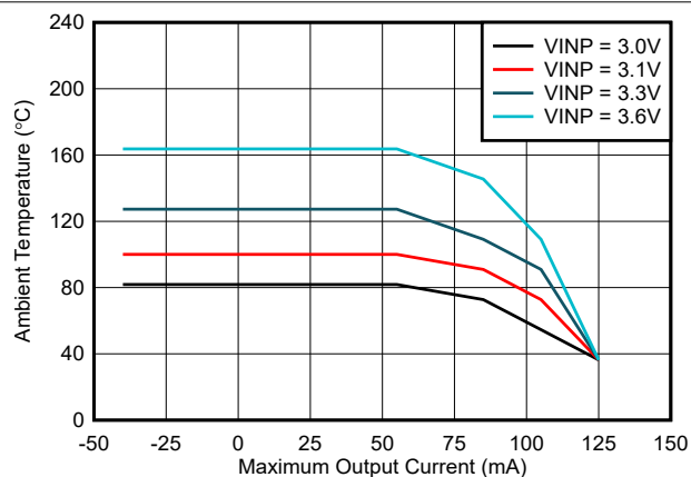
图 6-8. 最大输出电流与环境温度间的关系：VCC = 5.5V, COUT2 = 22 μF
