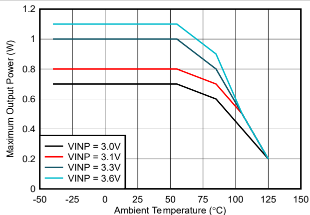
图 6-2. 最大输出功率与环境温度间的关系：VCC = 5.0V，COUT2 = 22 μF
