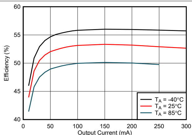
图 6-10. 效率与负载电流 ( I_{VCC} ) 间的关系：VCC = 5.0V, VINP = 5.0V, COUT2 = 22 μF
