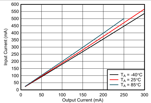
图 6-16. 输入电流 ( I_{VINP} ) 与负载电流 ( I_{VCC} ) 间的关系: V_{CC} = 5.0\text{V} , V_{INP} = 5.0\text{V} , C_{OUT2} = 22\text{ }\mu\text{F}
