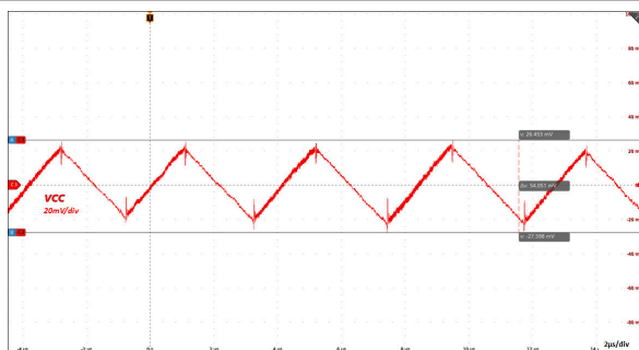
图 6-26. 稳态输出电压纹波 : VINP = 5.0V , VCC = 5.0V , C OUT2 = 22 µF , 300mA 负载
