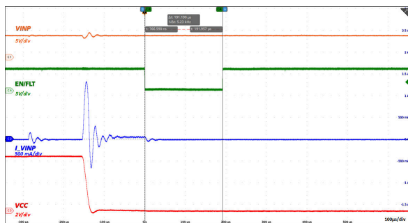
图 6-28. 输出短路运行 : VINP = 5.0V
