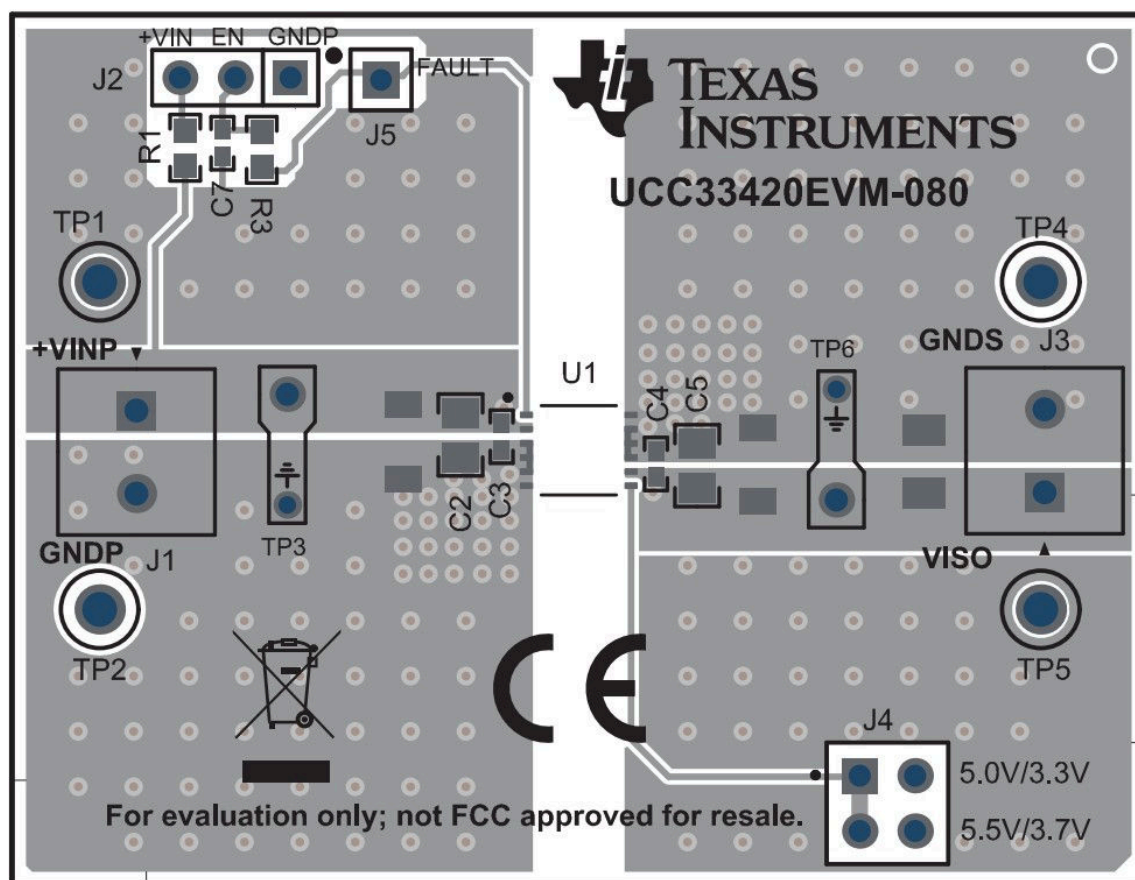
图 8-2. 布局示例
