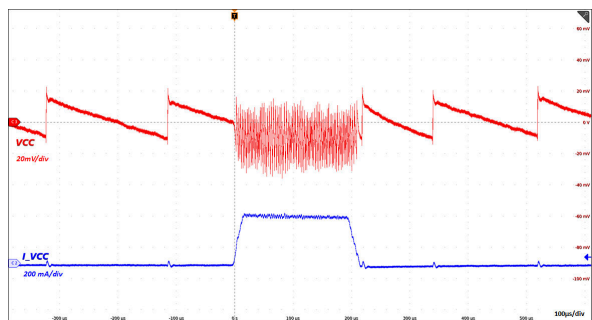
图 6-27. 负载瞬态 : VINP = 5.0V , VCC = 5.0V , C OUT2 = 22 µF , I VCC = 0mA - 300mA - 0mA
