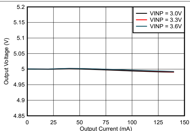
图 6-22. 输出电压调节 ( V_{VCC} ) 与负载电流 ( I_{VCC} ) 间的关系: V_{CC} = 5.0V , T_A = 25^\circ C , C_{OUT2} = 22 \mu F
