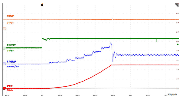
图 6-25. 通过 EN/FLT 从低电平到高电平启动 : VINP = 5.0V , VCC = 5.0V , 18Ω 负载
