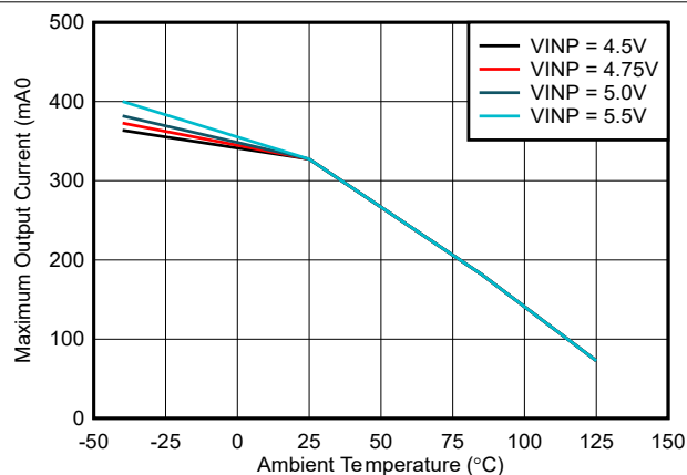
图 6-7. 最大输出电流与环境温度间的关系：VCC = 5.5V
