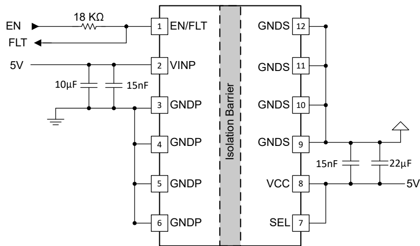
图 8-1. 典型应用
