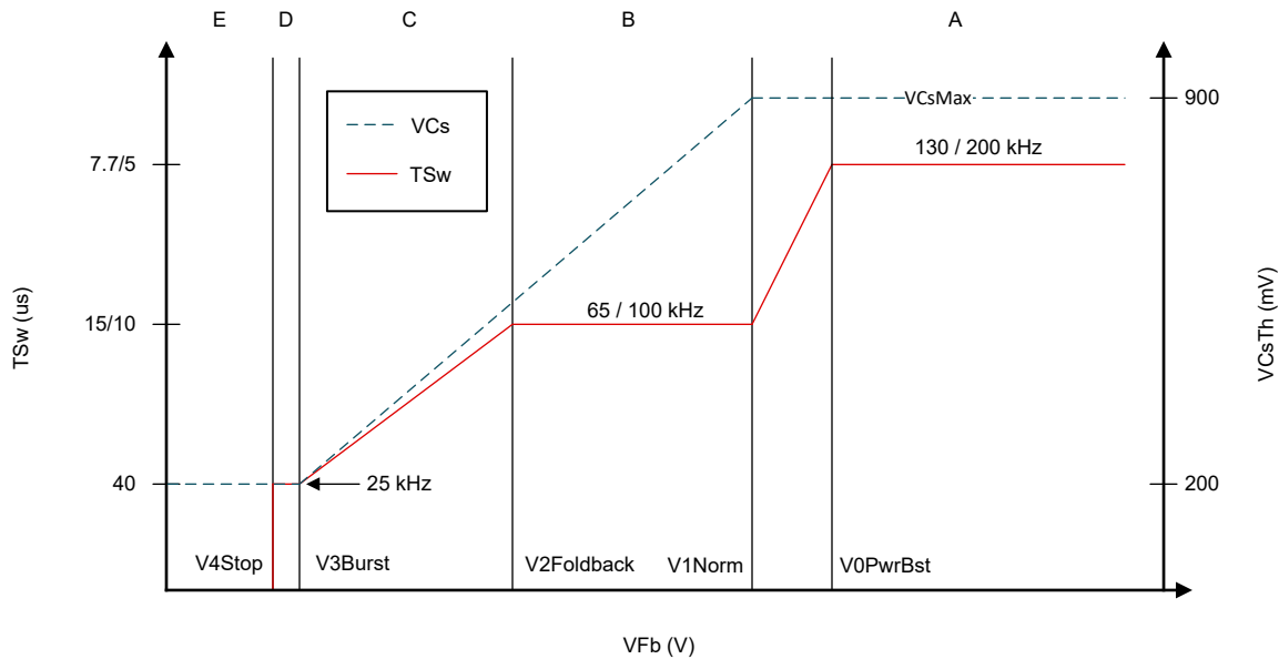
图 7-9. UCC28750 控制律
