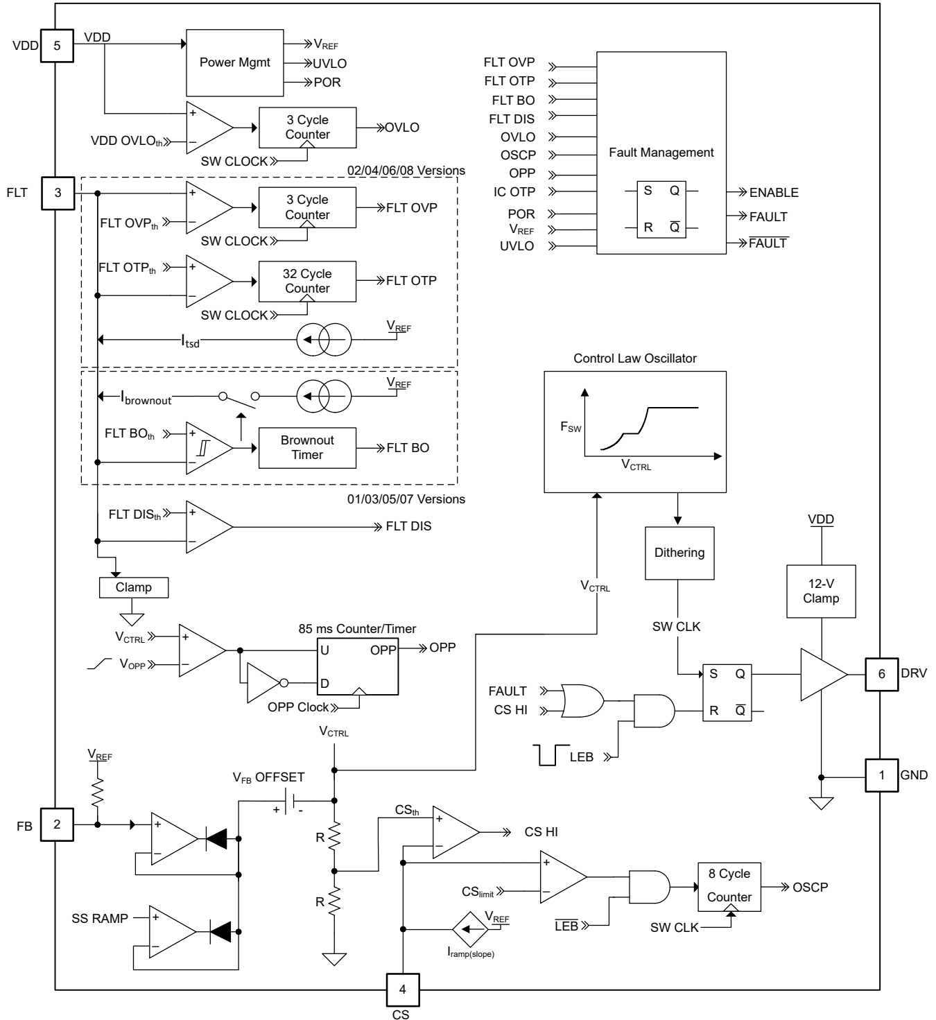
图 7-2. 功能方框图
