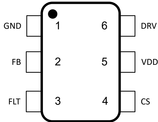
图 5-1. DBV 封装 (6 引脚) 俯视图
