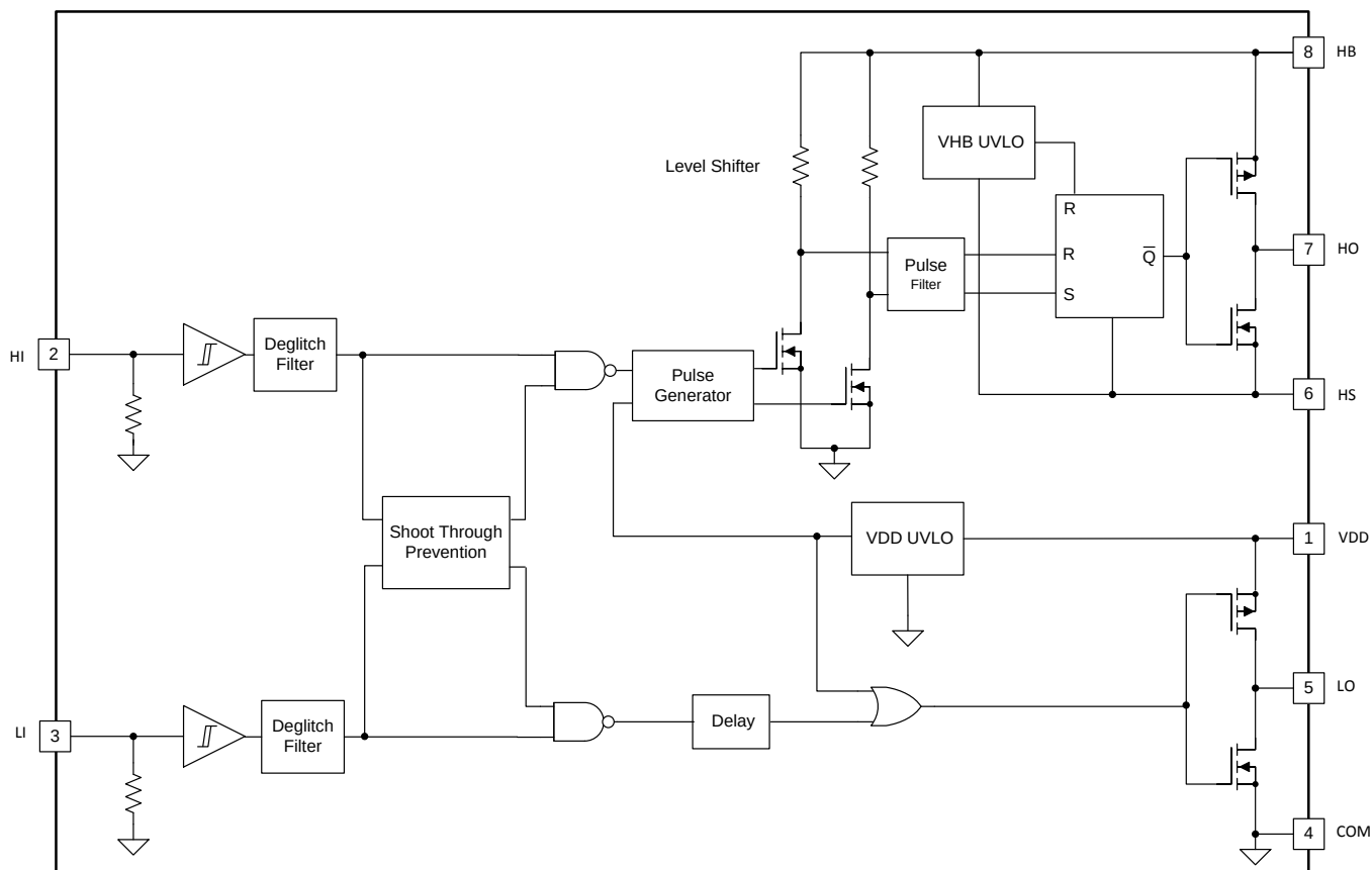
图 29. UCC27710 Block Diagram
