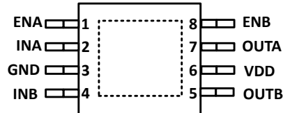
图 4-2. DGN 封装 8 引脚 VSSOP 顶视图
