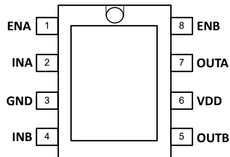
图 4-5. DDA 封装 8 引脚 SOIC 顶视图
