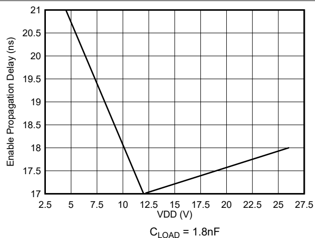
图 5-20. 使能到输出上传传播延迟
