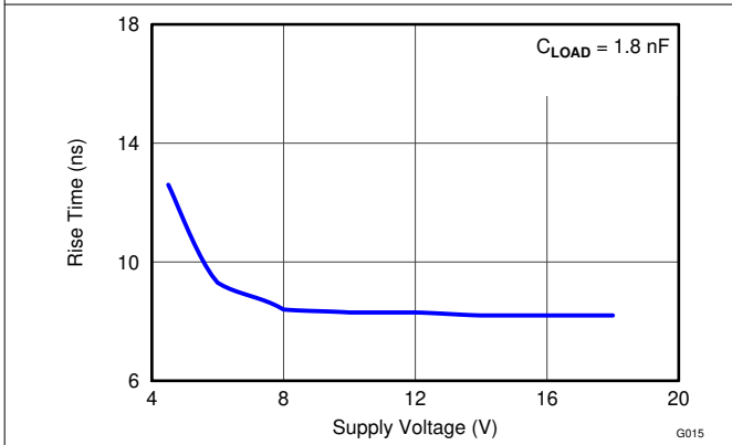
图 6-19. 上升时间与电源电压间的关系
