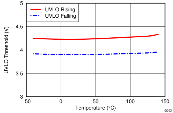
图 6-8. UVLO 阈值与温度间的关系
