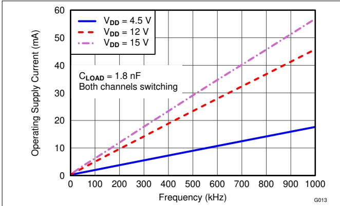
图 6-17. 工作电源电流与频率间的关系
