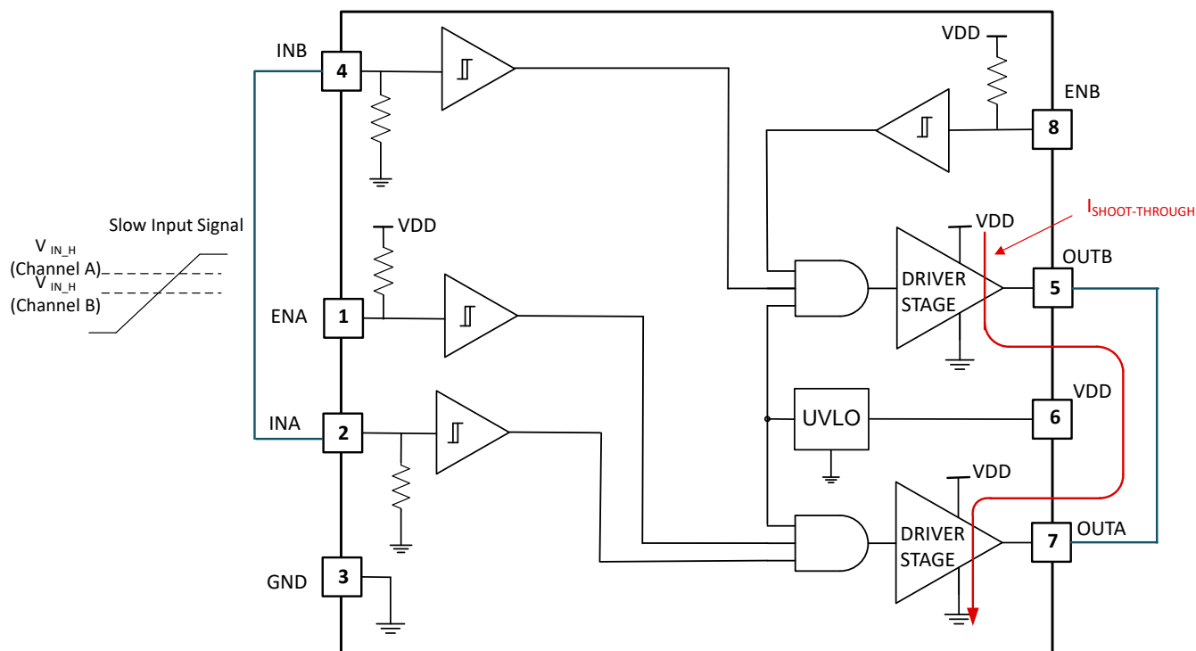
图 6-2. 慢速输入信号会在并联期间导致通道间出现击穿 ( 建议 dv/dt 为 20V/ms 或更高 )
