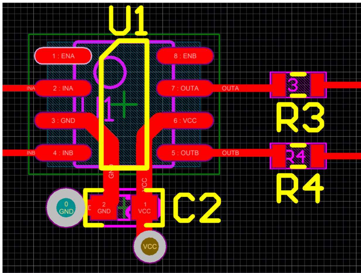
图 9-1. UCC27524A 布局示例
