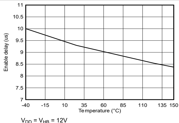
图 5-15. 启用延迟与温度间的关系
