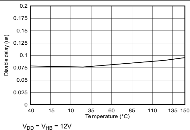
图 5-16. 禁用延迟与温度间的关系
