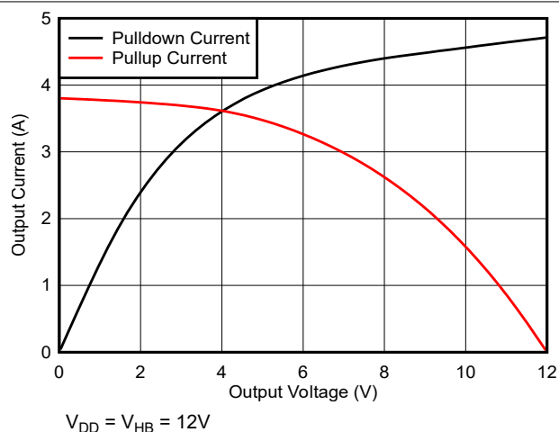
图 5-17. 输出电流与输出电压间的关系
