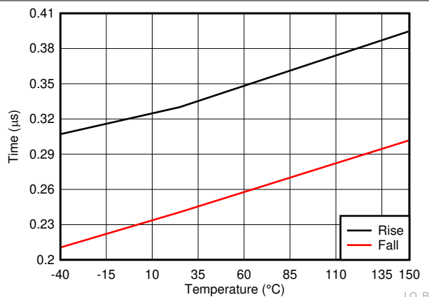
图 6-24. HO Rise Time
