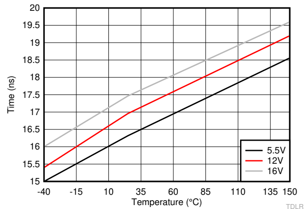
图 6-30. LO Rising Propagation Delay (TDLRR)
