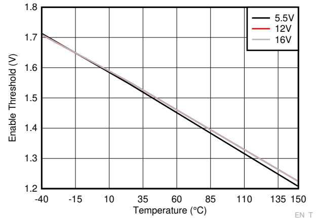
图 6-10. Enable Threshold
