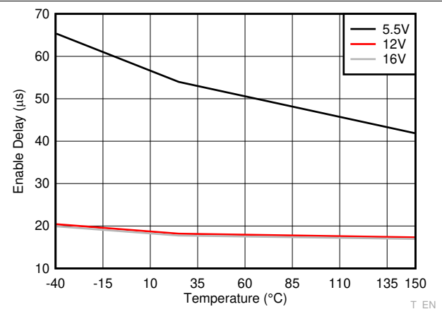
图 6-12. Enable Delay
