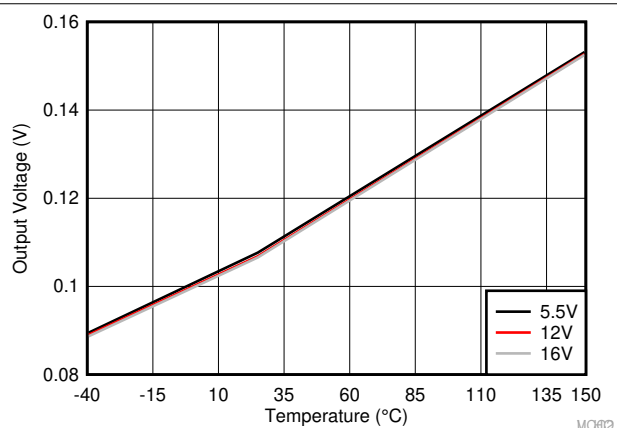
图 6-18. LO Low Output Voltage ( V_{LOL} )
