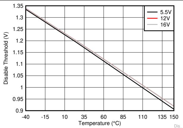
图 6-11. Disable Threshold
