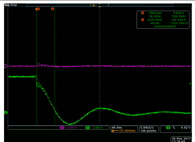
图 8-4. HO Fall Time
