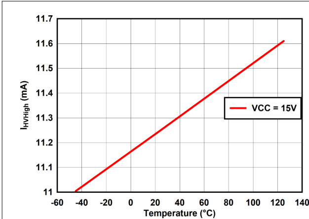
图 6-1. I_{HVHigh} 与温度间的关系
