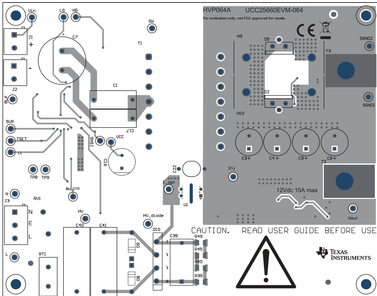
图 8-7. UCC25660EVM-064 ( 顶视图 )
