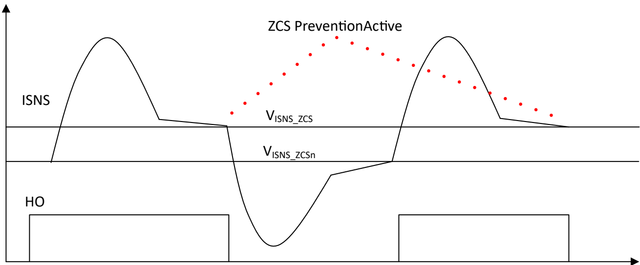
图 7-8. ZCS 保护
