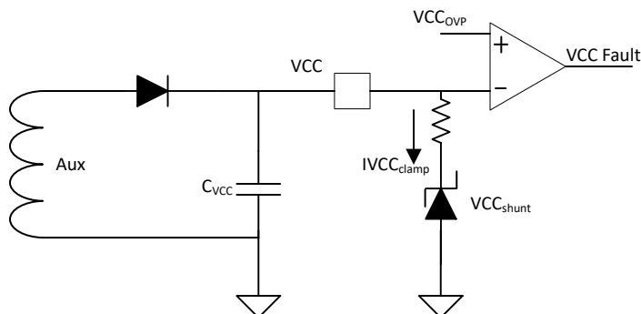
图 7-12. VCC 钳位
