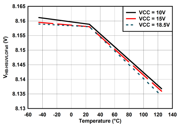
图 6-15. V_{HB-HSUUVLOFall} 与温度间的关系
