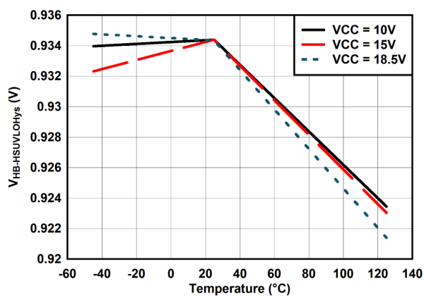
图 6-16. V_{HB-HSUUVLOHys} 与温度间的关系
