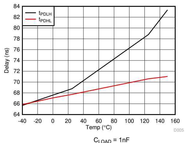
图 6-8. 传播延迟与温度间的关系
