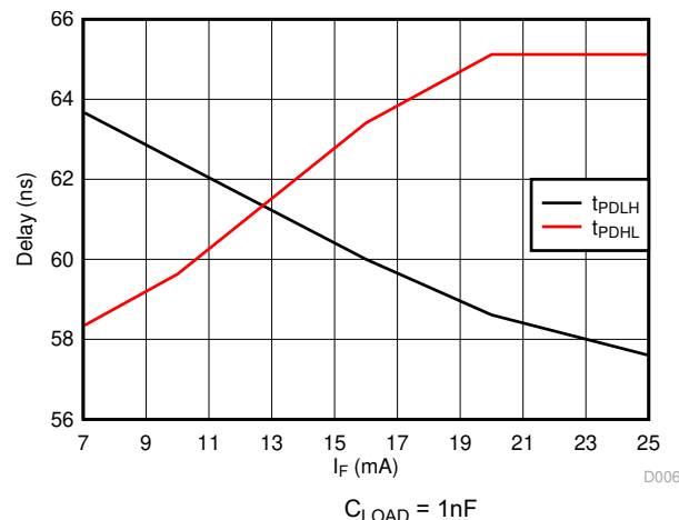
图 6-9. 传播延迟与正向电流间的关系
