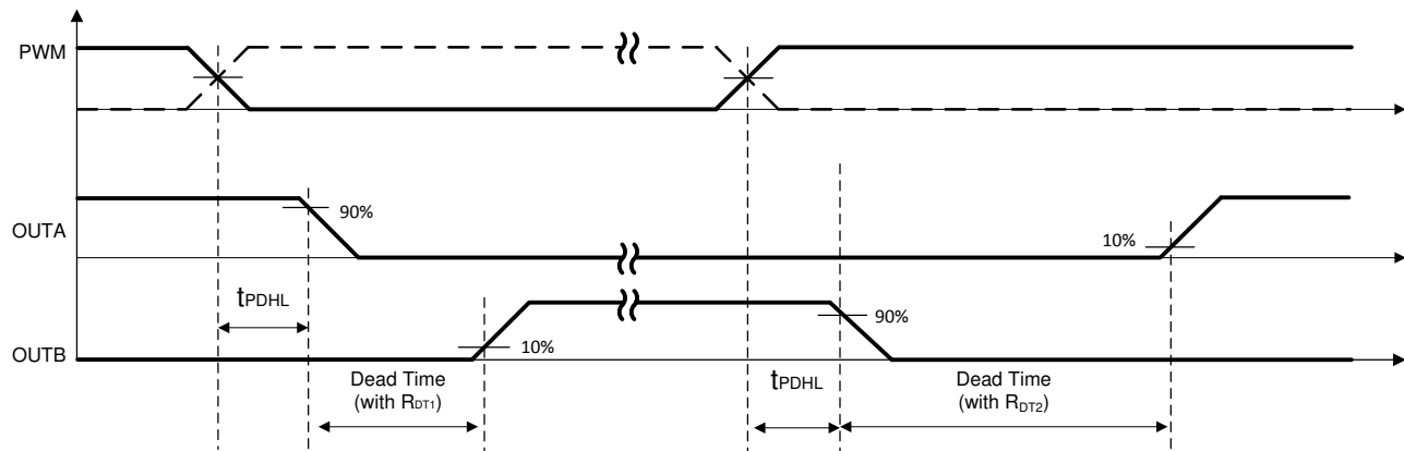
图 29. Dead-Time Switching Parameters
