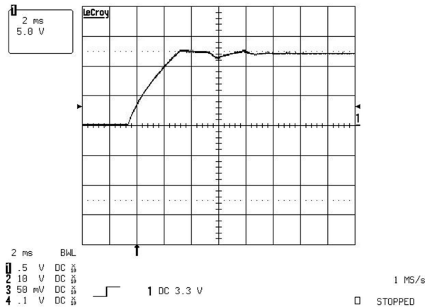
图 8-10. 满载启动条件下的输出电压行为 (5V/div)
