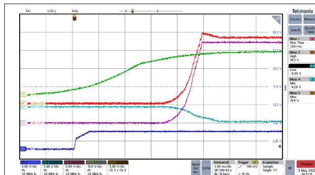
图 12-11. 上电序列。
