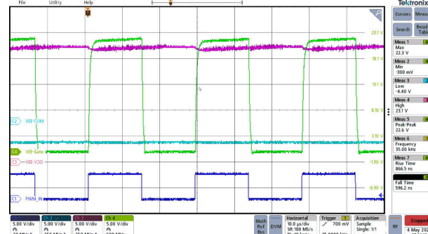
图 12-17. 在 35kHz 条件下开关 100nF 的栅极波形。
