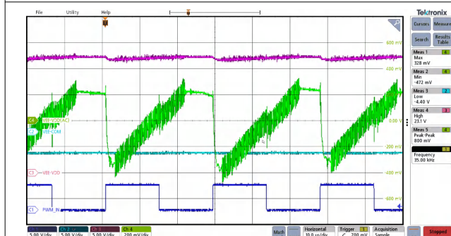
图 12-15. 纹波电压：VDD-VEE 在 35kHz 条件下开关 100nF 负载。
