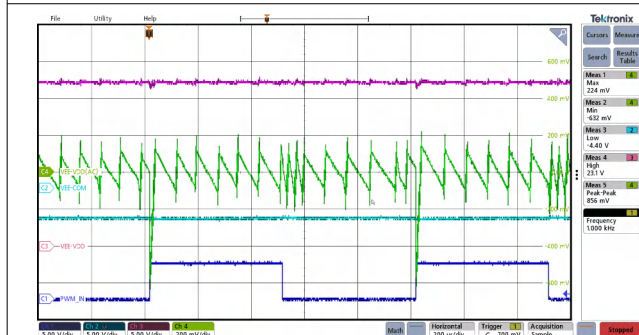
图 12-13. 纹波电压：VDD-VEE 在 1kHz 条件下开关 100nF 负载。
