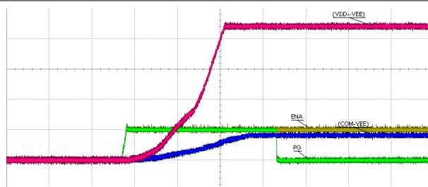
图 7-7. 启动: V_{IN} = 12\text{V} , V_{DD-VEE} = 22\text{V} , V_{COM-VEE} = 4\text{V} , V_{COM-VEE} 无负载。电压标度: 5V/div, 时间标度: 2ms/div。
