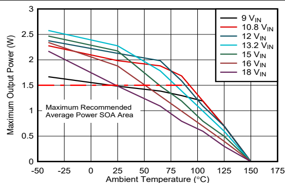
图 7-3. SOA 降额曲线: V_{DD-VEE} = 18\text{V} , V_{COM-VEE} = 3\text{V} , T_{shut} = 160^\circ\text{C} , V_{COM-VEE} 无负载
