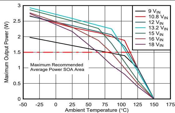
图 7-5. SOA 降额曲线: V_{DD-VEE} = 25\text{V} , V_{COM-VEE} = 5\text{V} , T_{shut} = 160^\circ\text{C} , V_{COM-VEE} 无负载
