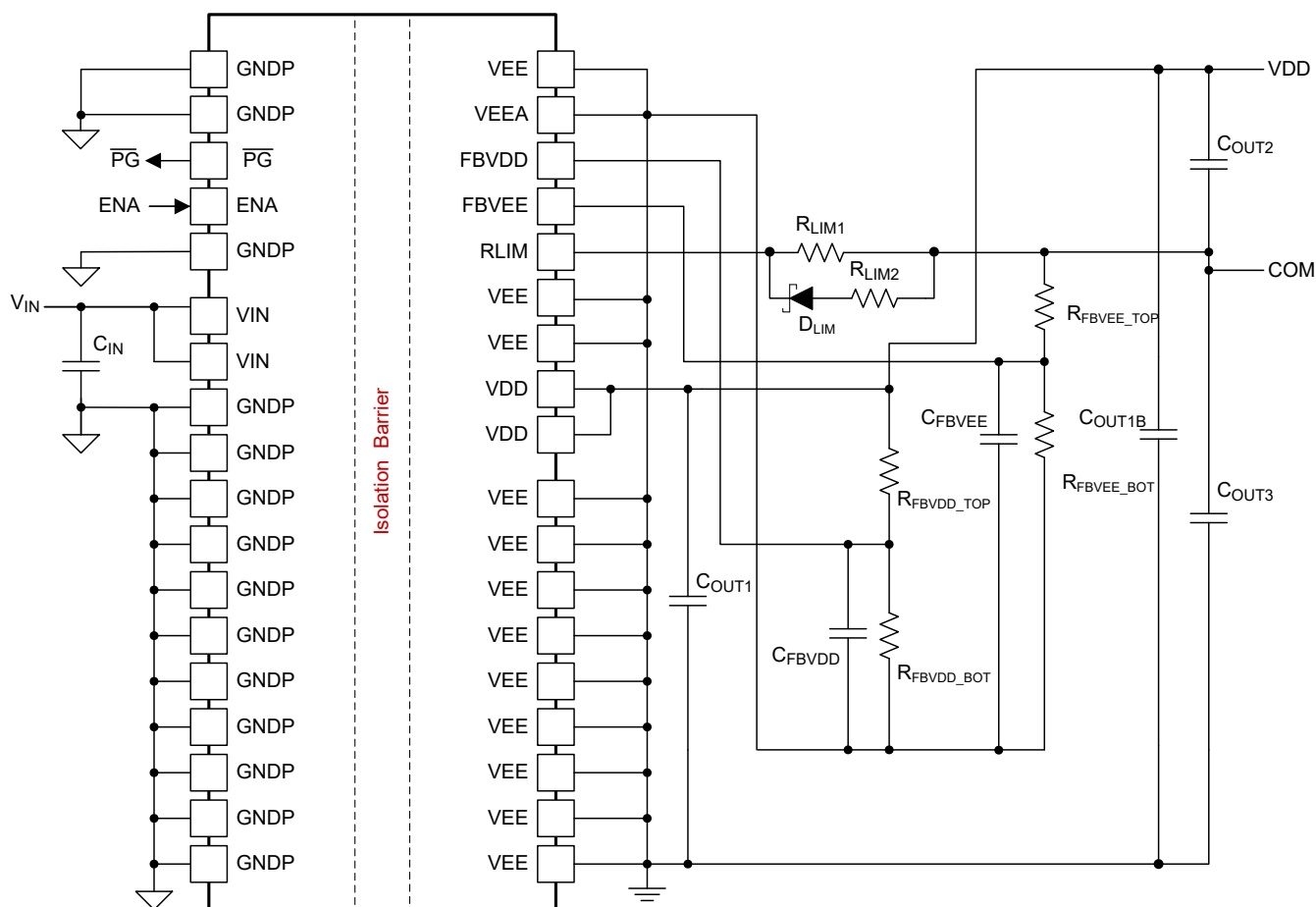
图 9-1. 双路可调输出配置
