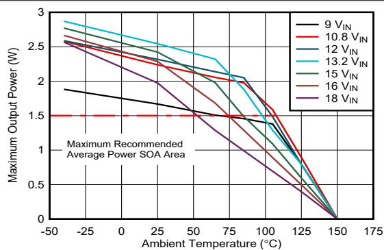
图 7-4. SOA 降额曲线: V_{DD-VEE} = 22\text{V} , V_{COM-VEE} = 4\text{V} , T_{shut} = 160^\circ\text{C} , V_{COM-VEE} 无负载
