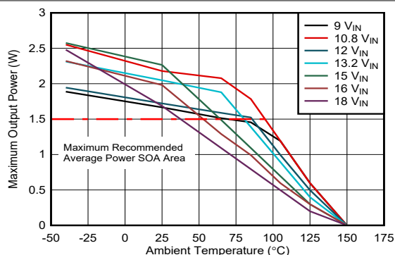
图 7-6. SOA 降额曲线: V_{DD-VEE} = 22\text{V} , V_{COM-VEE} = 4\text{V} , T_{shut} = 150^\circ\text{C} , V_{COM-VEE} 无负载, 在屏蔽盒中测试。
