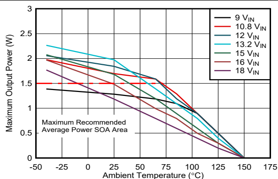
图 7-2. SOA 降额曲线: V_{DD-VEE} = 15\text{V} , V_{COM-VEE} = 5\text{V} , T_{shut} = 160^\circ\text{C} , V_{COM-VEE} 无负载
