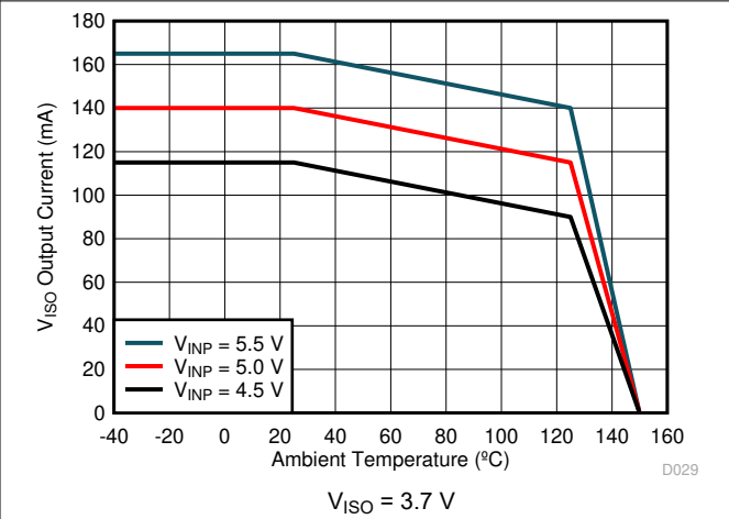
图 6-11. Maximum V_{ISO} Output Current vs. Temperature
