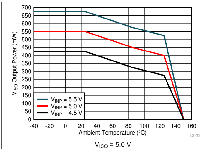
图 6-4. Maximum V_{ISO} Output Power vs. Temperature
