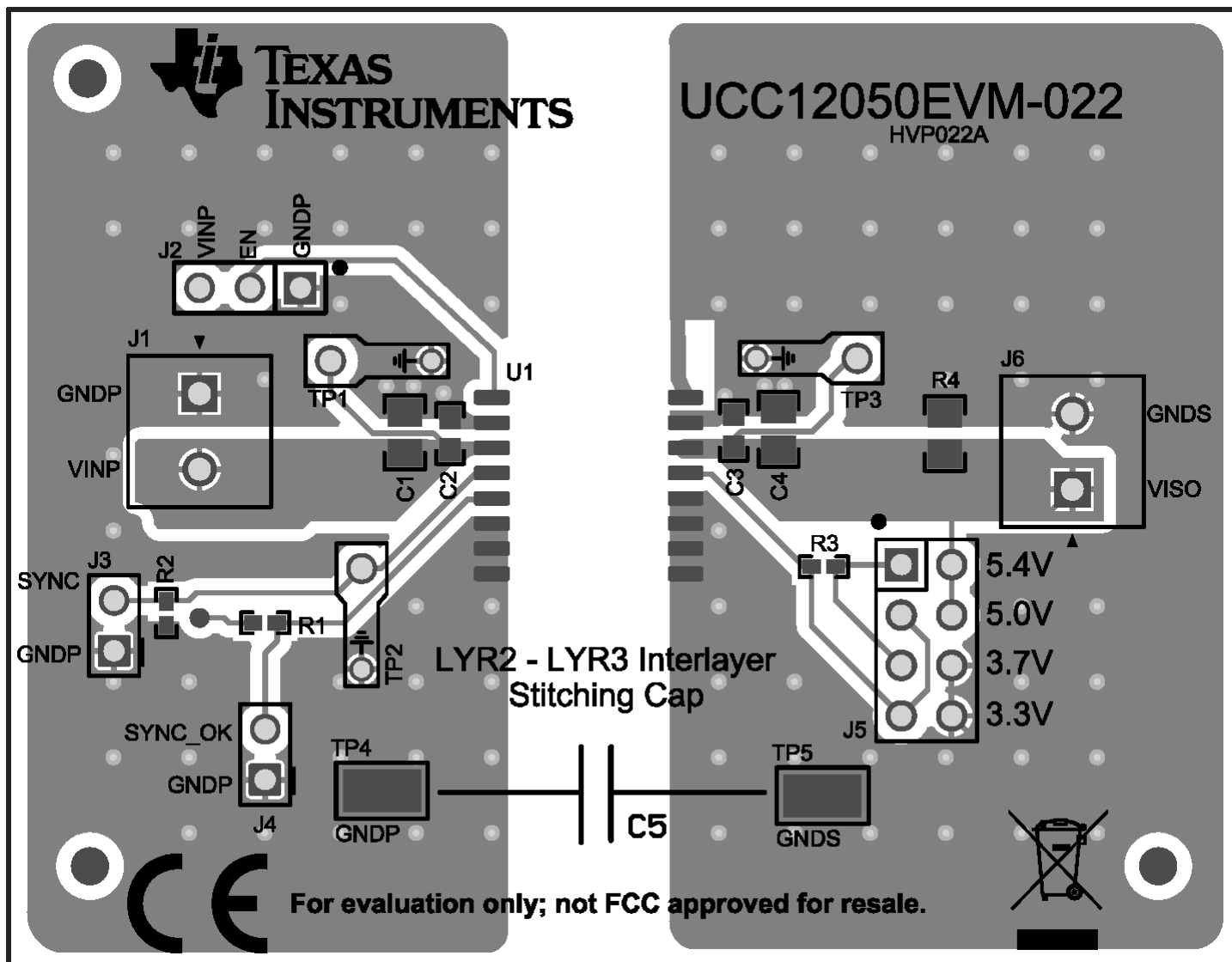
图 10-1. Layout Example
