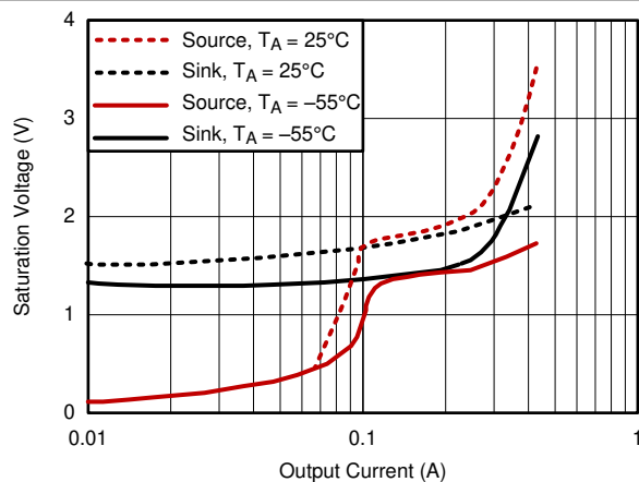
图 6-8. 输出饱和
