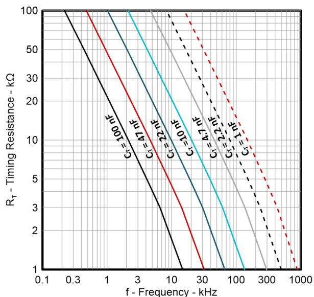
图 6-10. 时序电阻 R_{RT} 与频率间的关系
