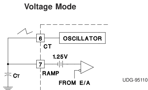
图 7-5. Control Methods
