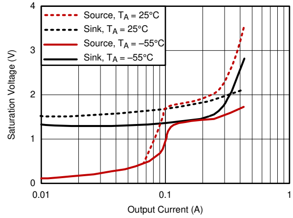
图 6-8. 输出饱和
