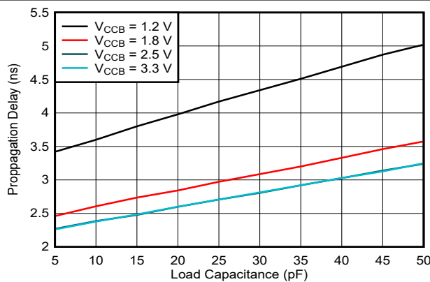
图 5-5. 传播延迟与负载电容间的关系 ( V_{CCA} = 1.2\text{V} )
