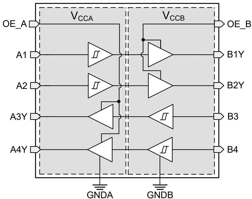
图 7-2. TXG1042-Q1 功能方框图
