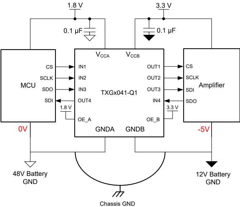
图 8-1. 汽车中的 TXG1041-Q1
