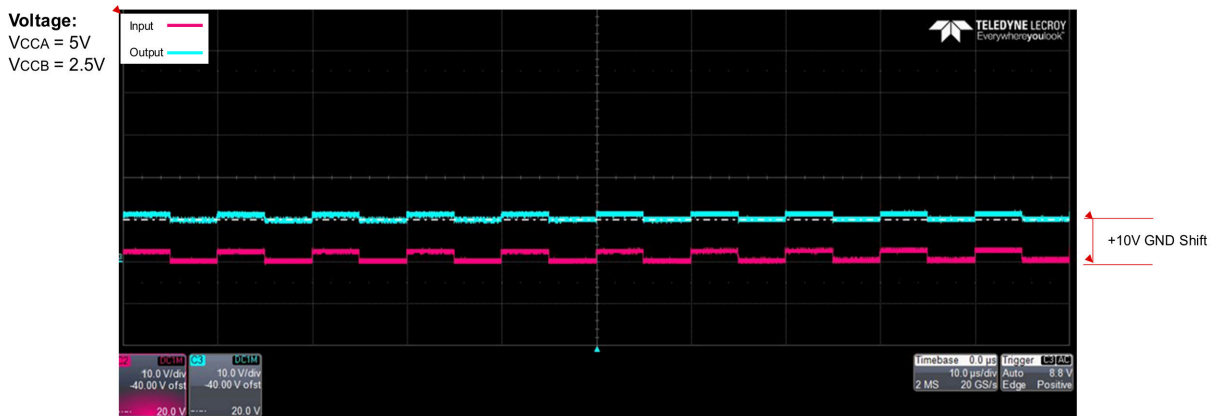
图 8-2. 显示了 5V 至 2.5V I/O 转换的 -10V (顶部) 和 +10V (底部) 接地漂移的波形
