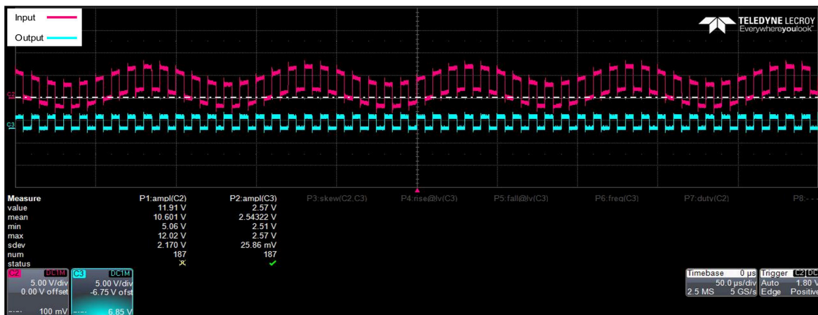
图 7-6. 显示了在交流接地噪声为 2V_{PP} (10kHz) 时 5V 至 2.5V I/O 转换的波形
