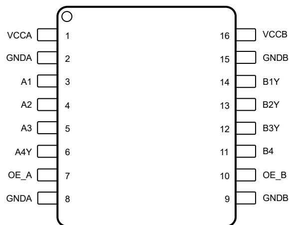
图 4-5. TXGx041DBQ 16 引脚 QSOP 顶视图
