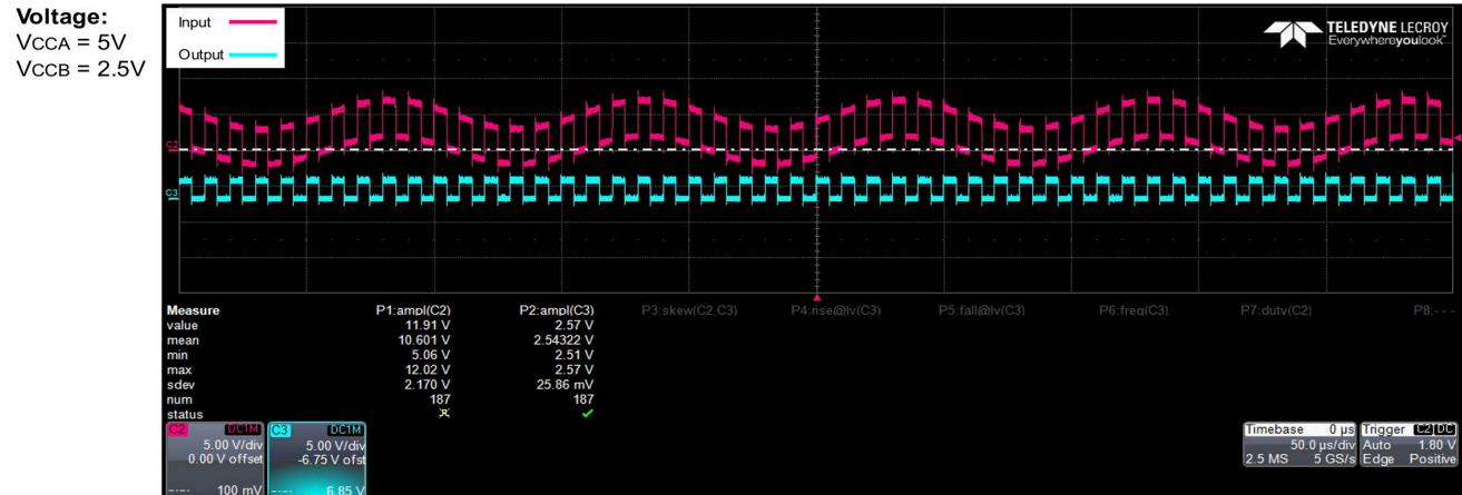
图 7-5. 显示了在交流接地噪声为 2V_{PP} (10kHz) 时 5V 至 2.5V I/O 转换的波形
