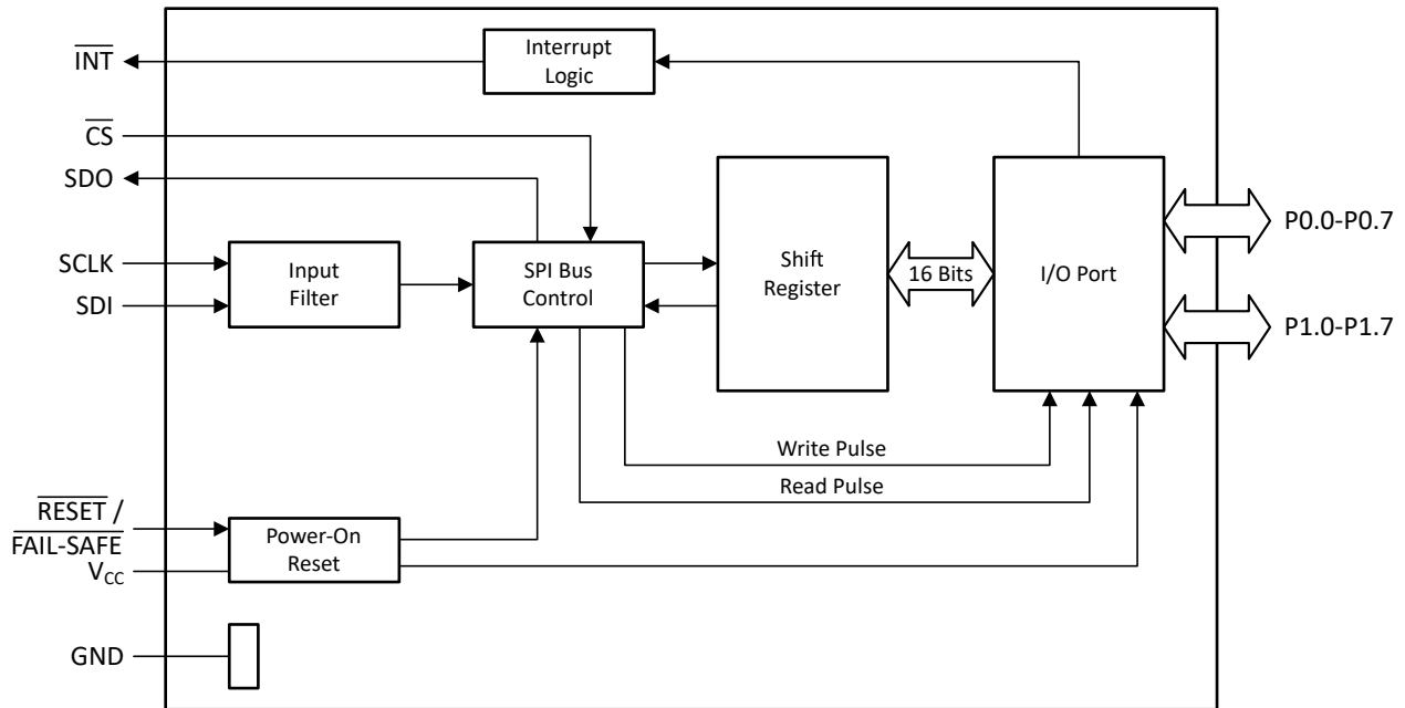
图 7-1. 逻辑图
