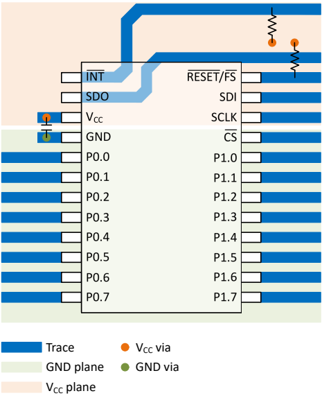
图 8-6. TXE8116-Q1 布局
