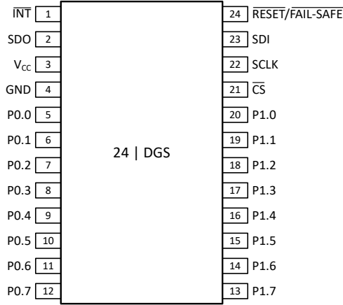
图 4-1. TXE8116-Q1 DGS (VSSOP) 封装，24 引脚 (顶视图)
