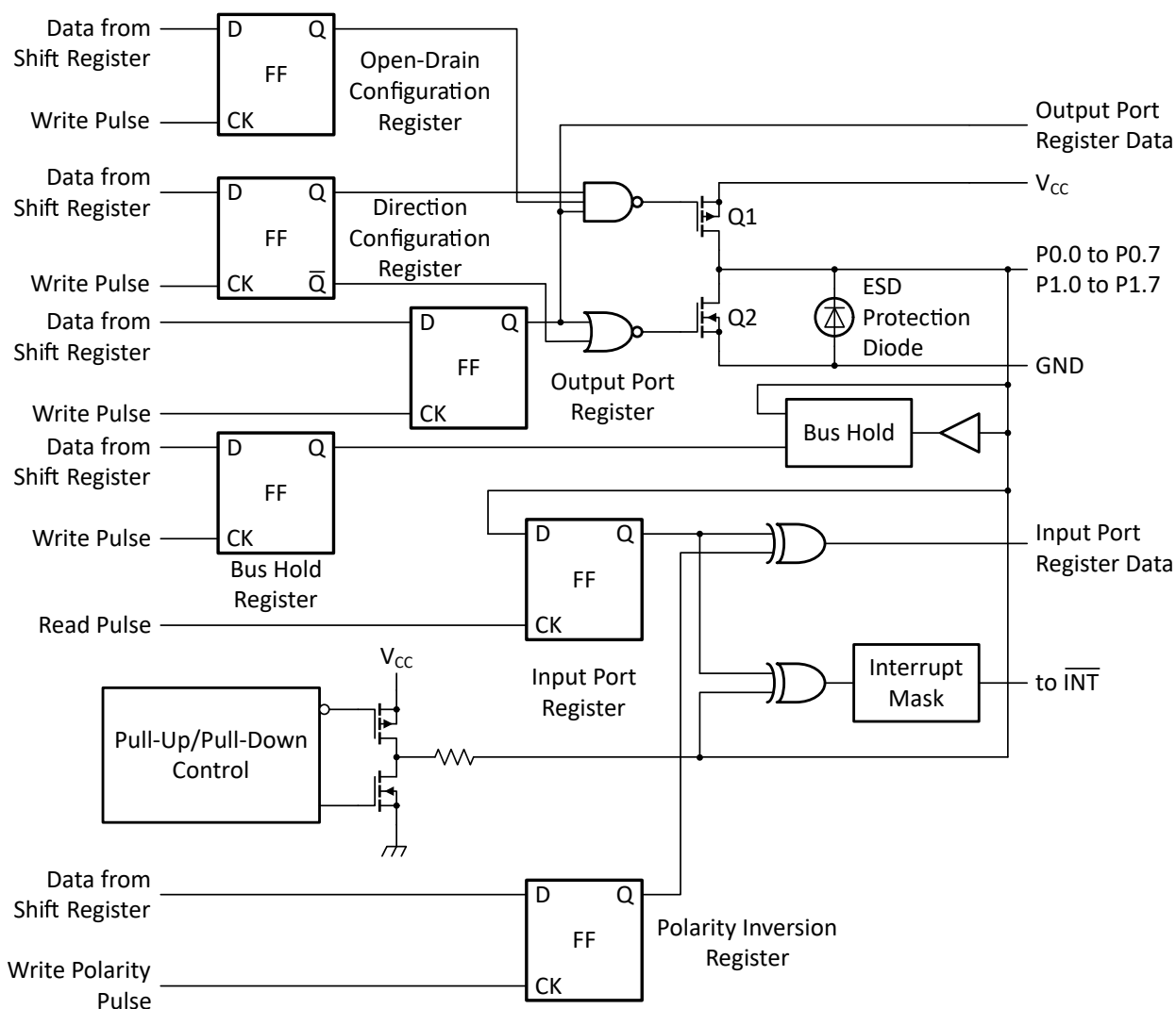
图 7-2. P0.0 至 P1.7 的简化版原理图
