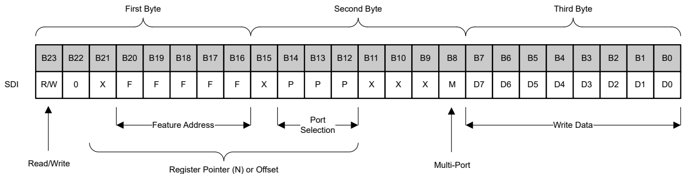
图 7-5. TXE8116-Q1 SPI SDI 数据帧格式
