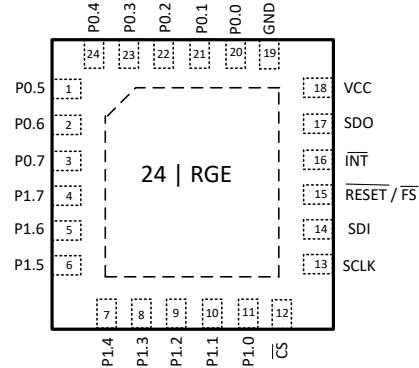
图 4-2. TXE8116-Q1 RGE (VQFN) 封装，24 引脚 (顶视图)
