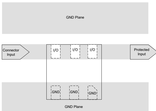
图 10-1. TVS5800 DFN1616 布局
