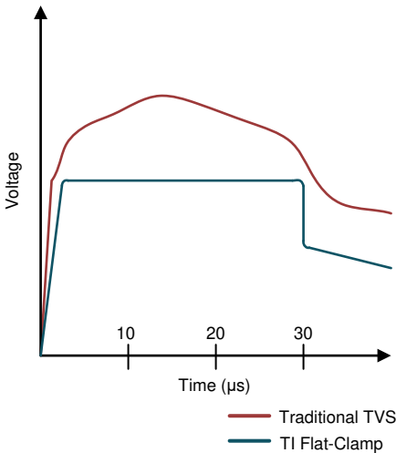
对 8/20μs 浪涌事件的电压钳位响应
