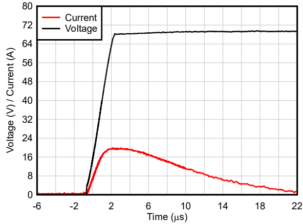
图 6-1. 电流为 20A 时，浪涌响应为 8/20 \mu\text{s}
