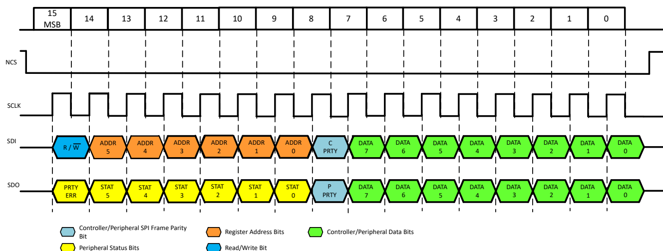
图 7-9. 16-Bit SPI Frame
