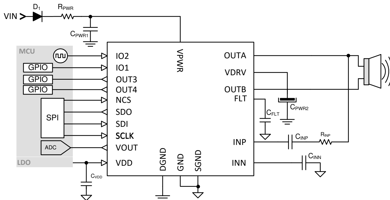
图 8-1. TUS4470 Application Diagram
