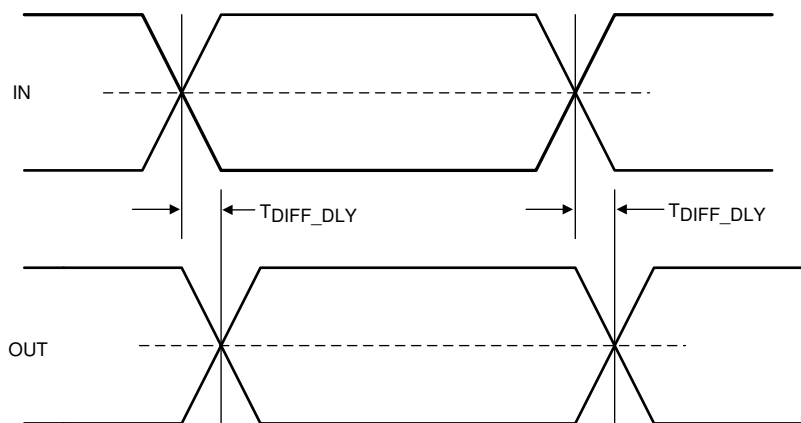
图 7-3. Propagation Delay
