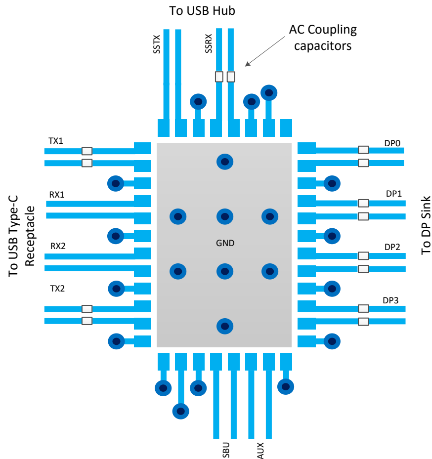
图 11-1. Layout Example
