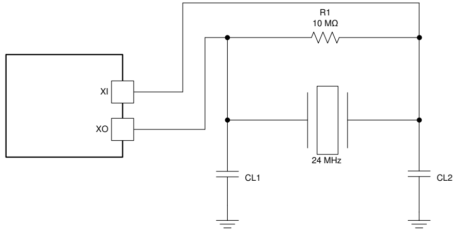
图 6-1. TUSB4041I 时钟
