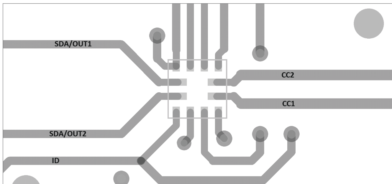
图 10-1. TUSB320 Layout
