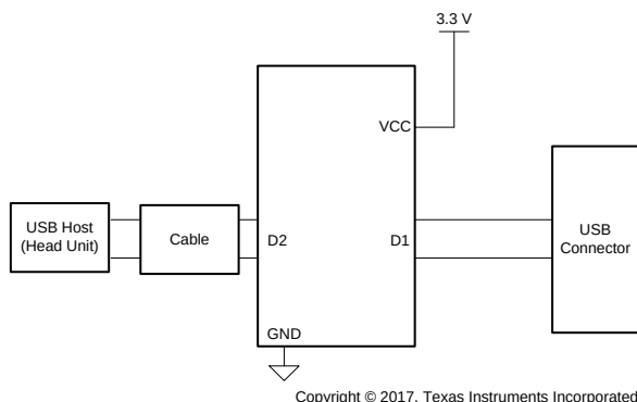
简化电路原理图
