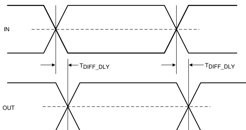
图 5-3. Propagation Delay
