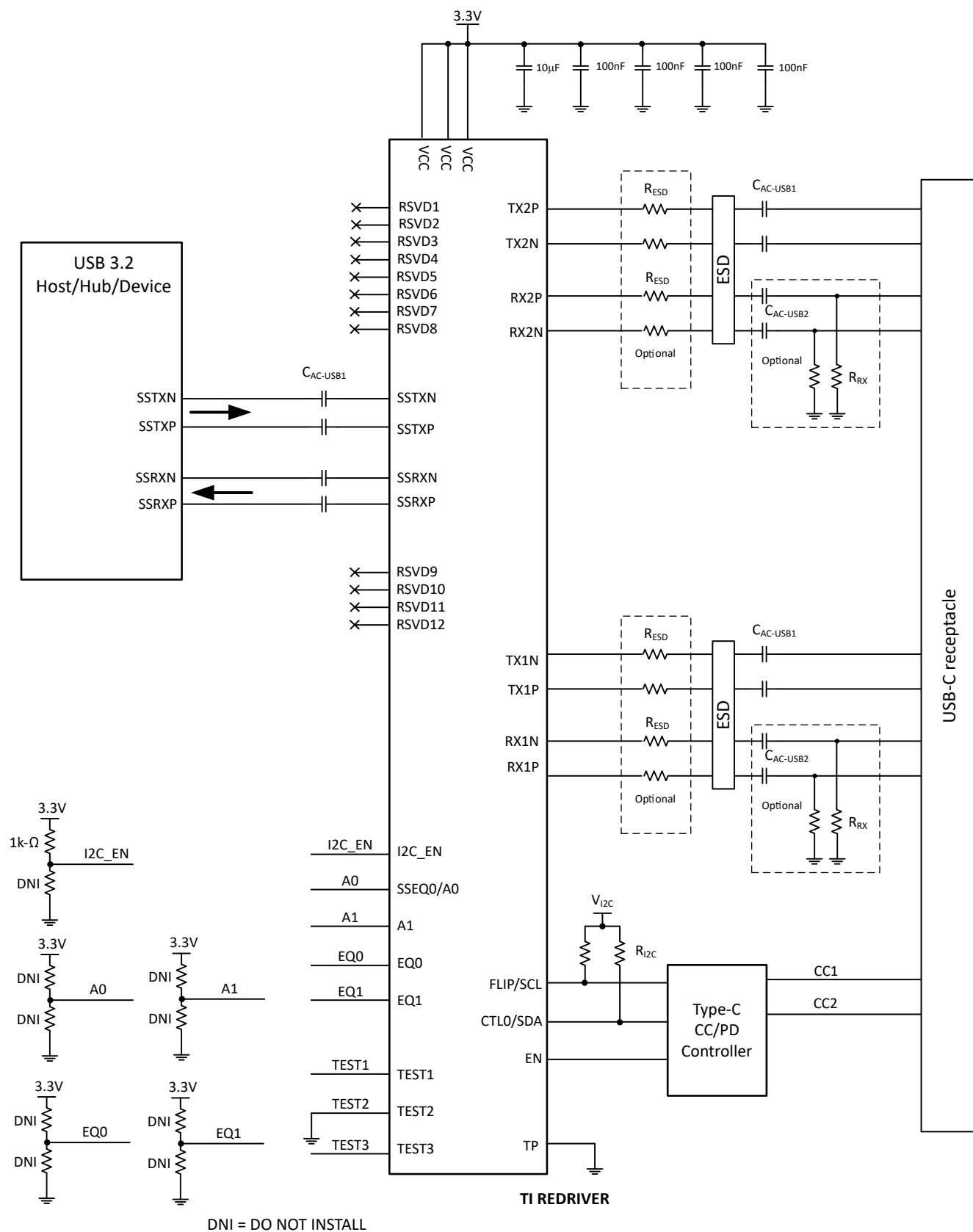
图 8-2. 应用电路
