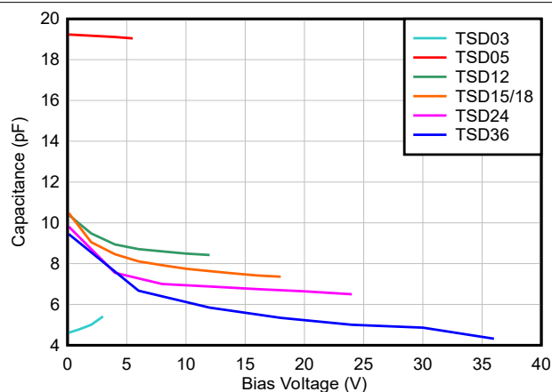
图 5-9. 电容与偏置电压之间的关系
