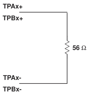
图 8-1. Test Load Diagram
