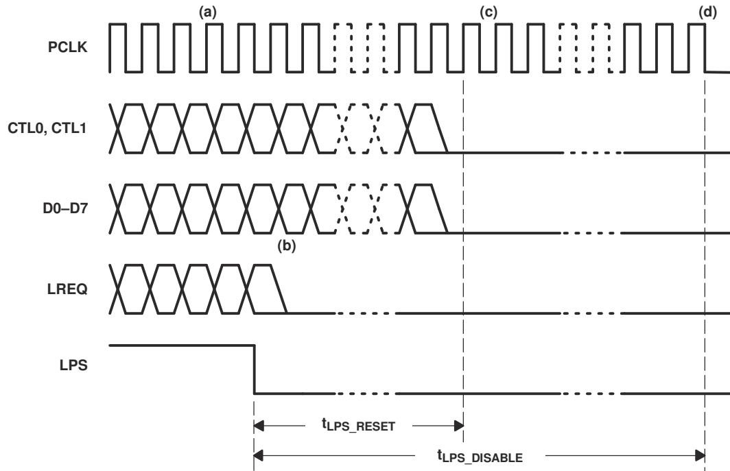
图 12-8. Interface Disable
