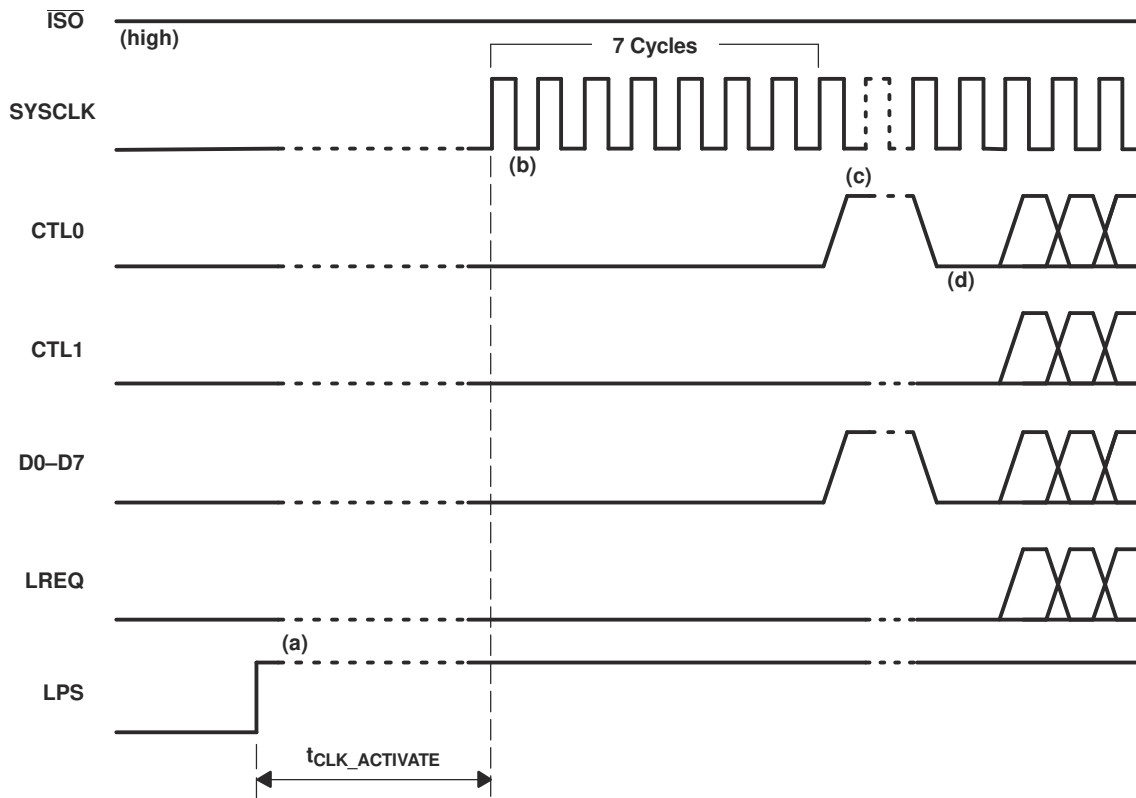
图 12-9. Interface Initialization
