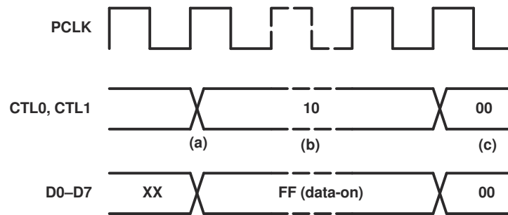
图 11-7. Null Packet Reception Timing
