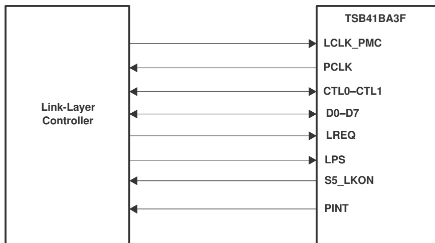
图 11-1. PHY-LLC Interface
