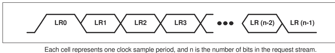
图 11-2. LREQ Request Stream
