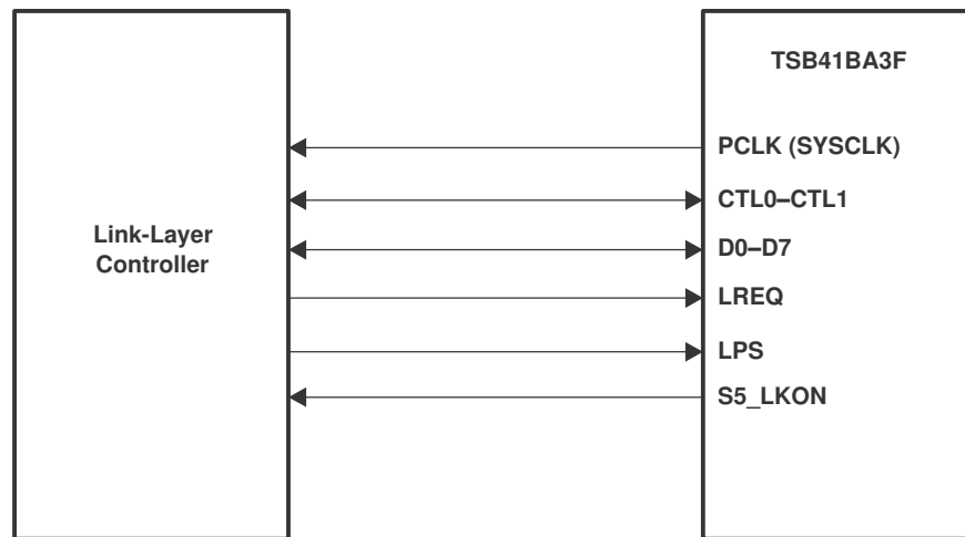
图 12-1. PHY-LLC Interface
