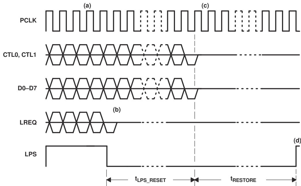
图 12-7. Interface Reset
