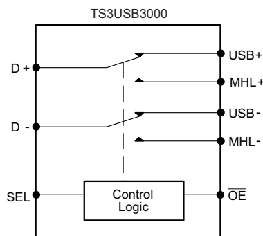
功能方框图
