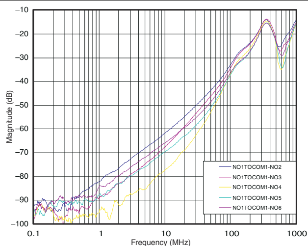
图 6-7. Crosstalk Adjacent
