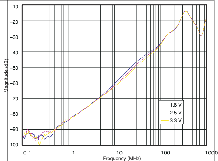
图 6-8. Crosstalk
