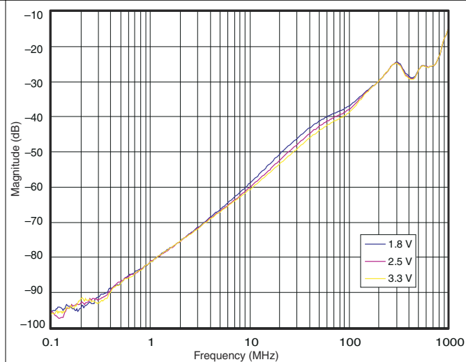
图 6-10. OFF Isolation
