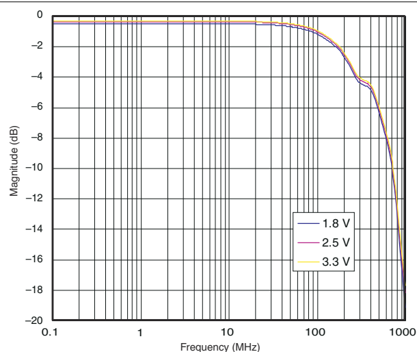
图 6-11. Insertion Loss
