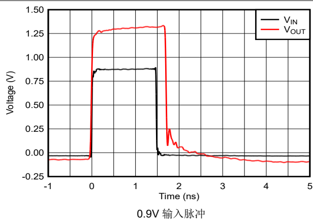
图 5-48. 过载恢复
