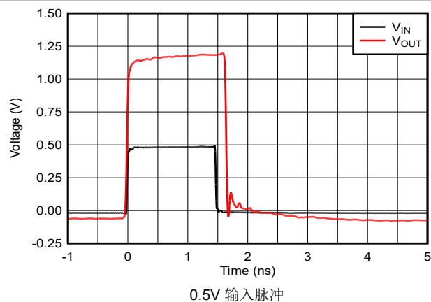
图 5-47. 过载恢复
