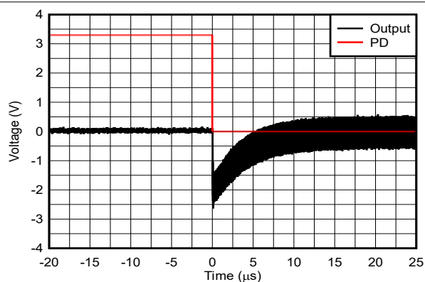
f = 500\text{MHz} , 100\text{nF} 交流耦合电容器
