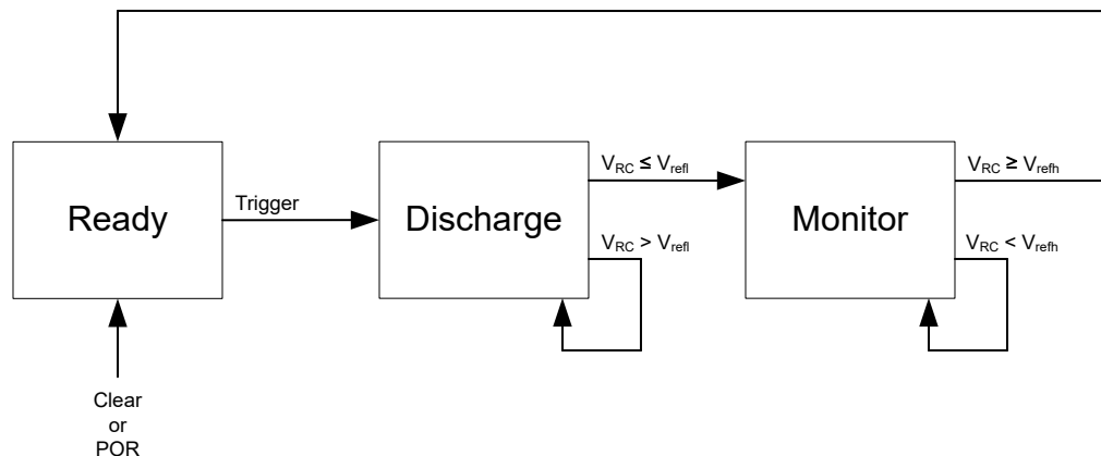
图 7-2. 状态机图
