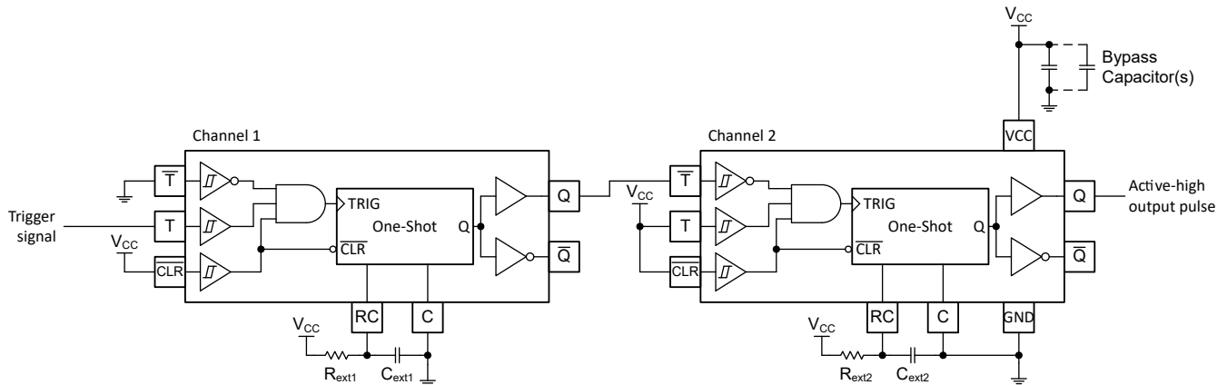
图 8-4. 使用 TPUL2T223 的延迟脉冲发生原理图
