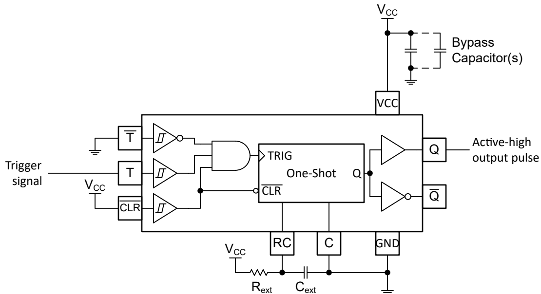
图 8-1. 使用 TPUL2T223 的脉冲发生器原理图
