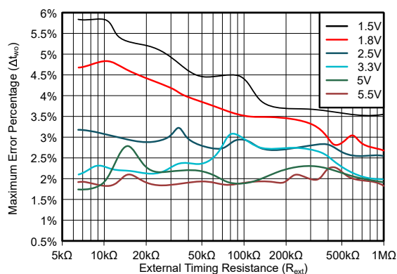
图 5-23. C_{ext} = 1\text{nF} 时最大输出脉冲宽度误差 (绝对值) 与时序电阻器值间的关系
