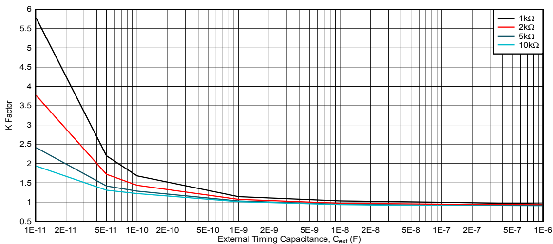
图 5-13. K 系数, V_{CC} = 3.3V , R_{ext} = 1k\Omega 至 10k\Omega
