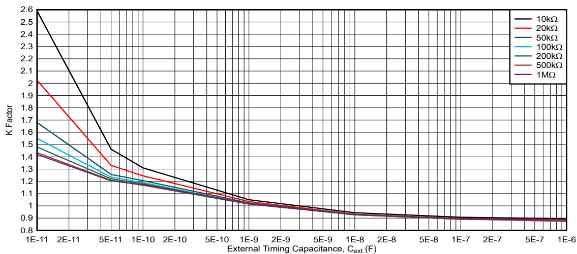
图 5-10. K 系数, V_{CC} = 1.8V , R_{ext} = 10k\Omega 至 1M\Omega
