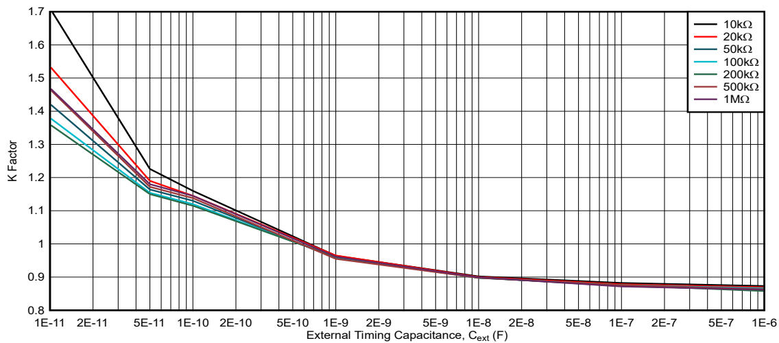
图 5-18. K 系数, V_{CC} = 5.5V , R_{ext} = 10k\Omega 至 1M\Omega
