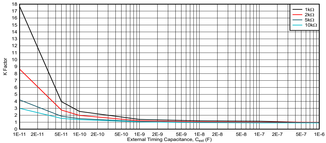
图 5-7. K 系数, V_{CC} = 1.5V , R_{ext} = 1k\Omega 至 10k\Omega
