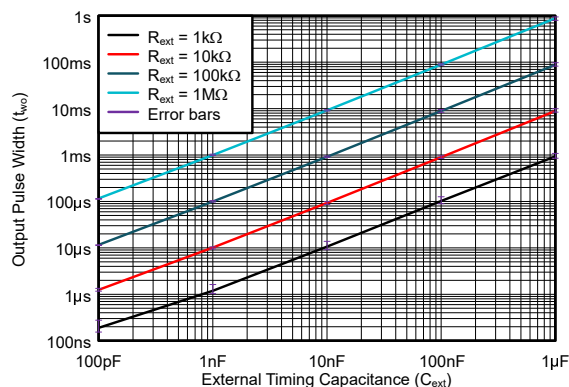
图 5-21. 典型输出脉冲宽度与时序电容值间的关系 ( 叠加误差栏 )
