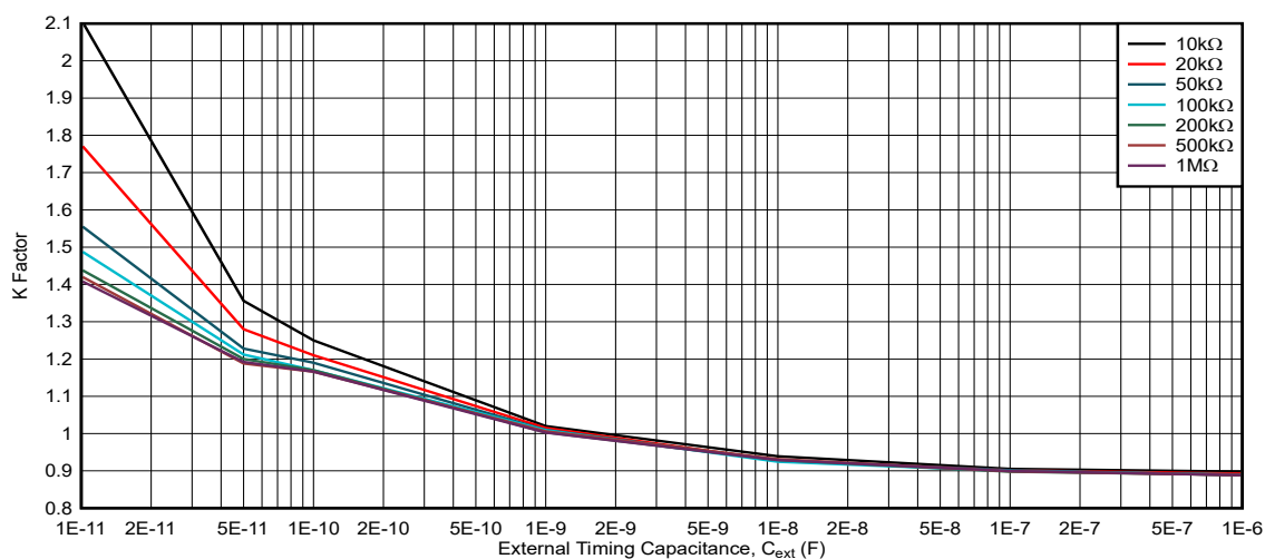
图 5-12. K 系数, V_{CC} = 2.5V , R_{ext} = 10k\Omega 至 1M\Omega
