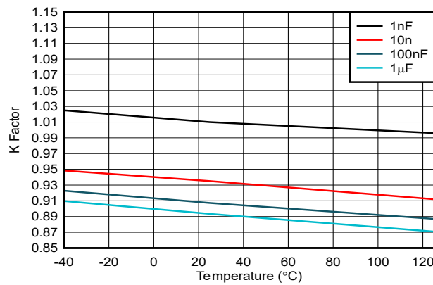
图 5-5. K 系数与温度间的关系, R_{ext} = 10k\Omega
