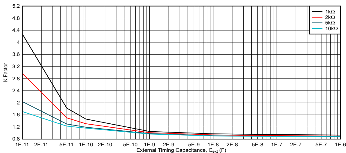
图 5-17. K 系数, V_{CC} = 5.5V , R_{ext} = 1k\Omega 至 10k\Omega
