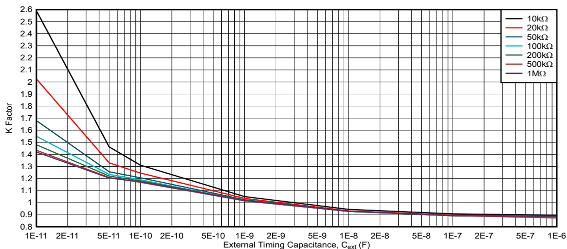
图 5-10. K 系数, V_{CC} = 1.8V , R_{ext} = 10k\Omega 至 1M\Omega
