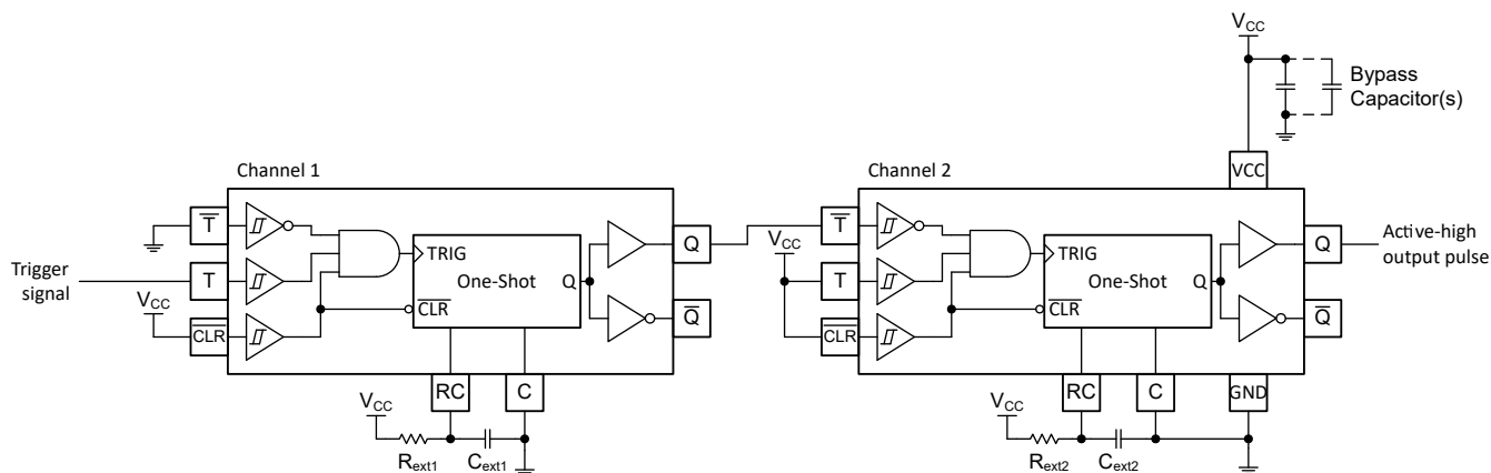
图 8-4. 使用 TPUL2T123 的延迟脉冲发生原理图
