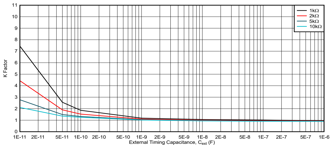
图 5-11. K 系数, V_{CC} = 2.5V , R_{ext} = 1k\Omega 至 10k\Omega
