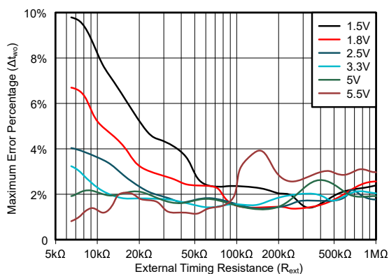
图 5-23. C_{ext} = 100\text{pF} 时最大输出脉冲宽度误差 ( 绝对值 ) 与时序电阻器值间的关系
