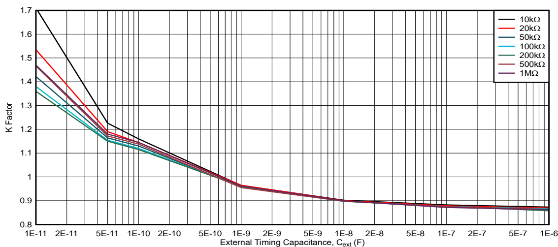
图 5-18. K 系数, V_{CC} = 5.5V , R_{ext} = 10k\Omega 至 1M\Omega
