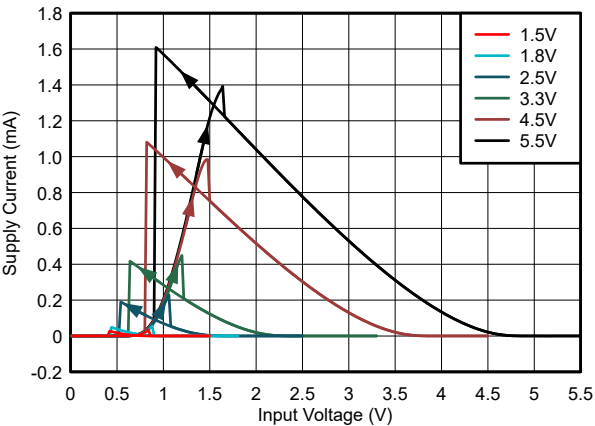
图 5-2. 电源电流与输入电压间的关系
