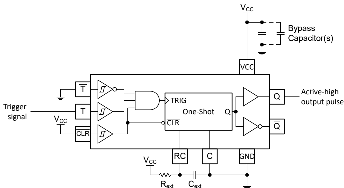
图 8-1. 使用 TPUL2T123 的脉冲发生器原理图
