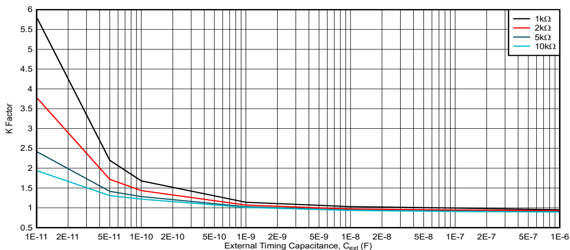
图 5-13. K 系数, V_{CC} = 3.3V , R_{ext} = 1k\Omega 至 10k\Omega
