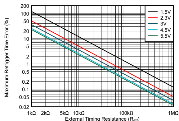
图 5-20. 最大重触发时间误差 (占总脉冲宽度的百分比) 与外部时序电阻器值间的关系
