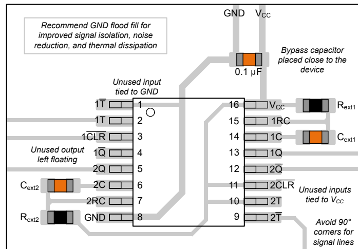
图 8-6. 采用 PW (TSSOP) 封装的 TPUL2T123 布局示例
