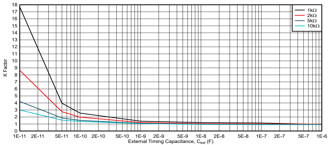
图 5-7. K 系数, V_{CC} = 1.5V , R_{ext} = 1k\Omega 至 10k\Omega
