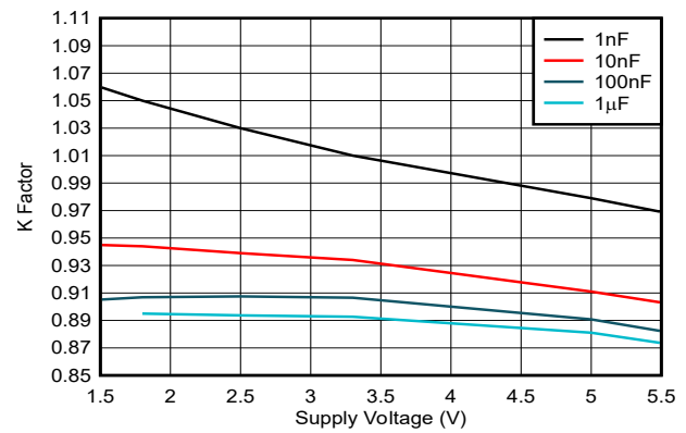
图 5-6. K 系数与电源电压间的关系, R_{ext} = 10k\Omega
