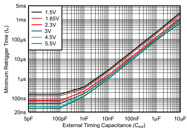
图 5-19. 最短重触发时间与外部时序电容器值间的关系
