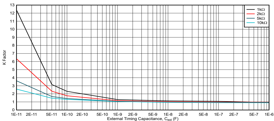
图 5-9. K 系数, V_{CC} = 1.8V , R_{ext} = 1k\Omega 至 10k\Omega
