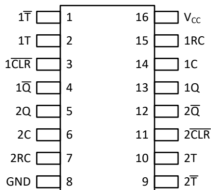
图 4-1. D、PW 封装 16 引脚 SOIC、TSSOP 顶视图
