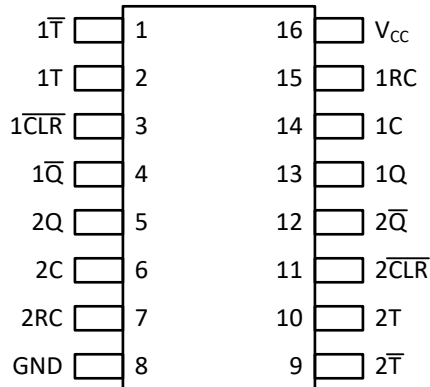
图 4-1. TPUL2T122-Q1 D 和 PW 封装 16 个引脚 SOIC 和 TSSOP 顶视图
