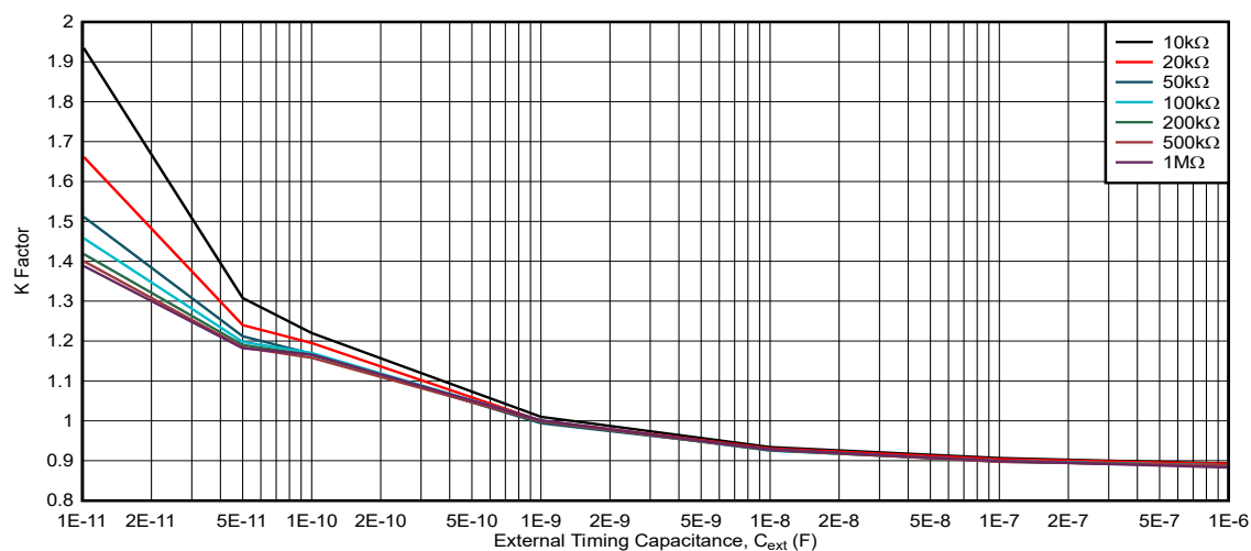
图 5-15. K 系数, V_{CC} = 3.3V , R_{ext} = 10k\Omega 至 1M\Omega
