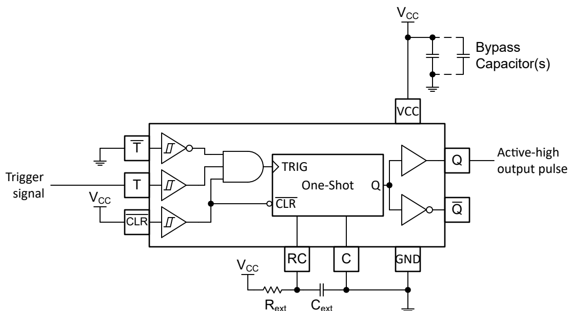
图 8-1. 使用 TPUL2T122x-Q1 的脉冲发生器原理图
