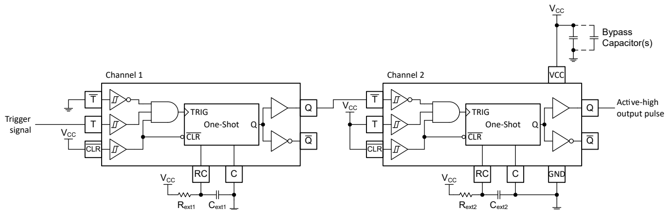
图 8-4. 使用 TPUL2T122x-Q1 的延迟脉冲发生原理图
