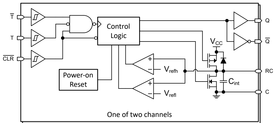
图 7-4. TPUL2T122A-Q1
