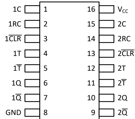
图 4-2. TPUL2T122A-Q1 D 和 PW 封装 16 个引脚 SOIC 和 TSSOP 顶视图
