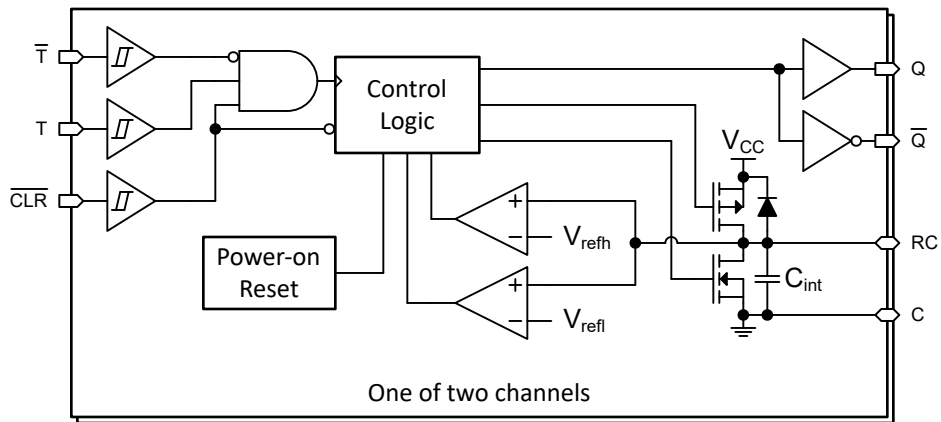
图 7-3. TPUL2T122-Q1
