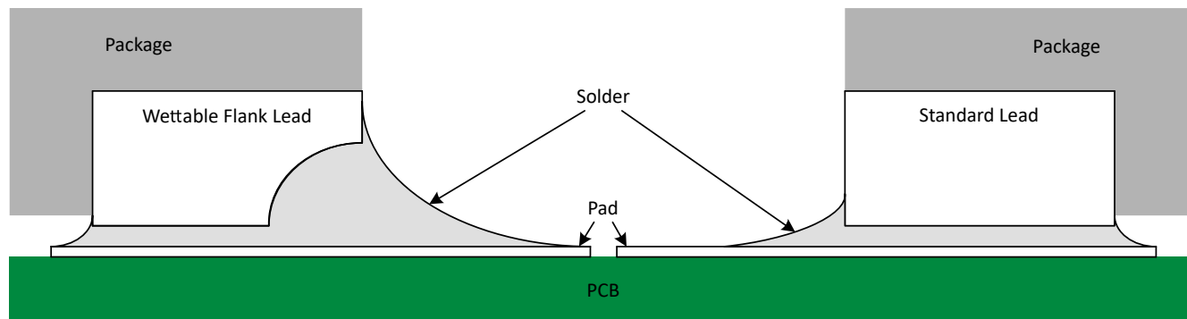
图 7-8. 焊接后具有可润湿侧翼的 QFN 封装和标准 QFN 封装的简化剖面图
