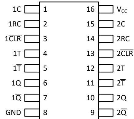
图 4-2. TPUL2G122A D 和 PW 封装 16 个引脚 SOIC 和 TSSOP 顶视图
