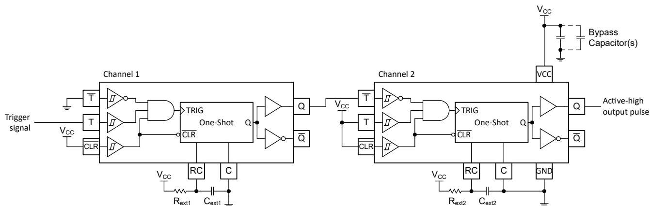
图 8-4. 使用 TPUL2G122x 的延迟脉冲发生原理图
