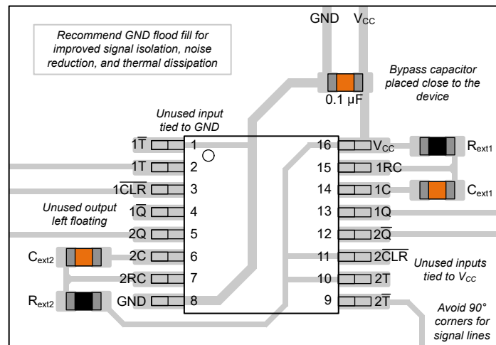
图 8-6. 采用 PW (TSSOP) 封装的 TPUL2G122x 布局示例
