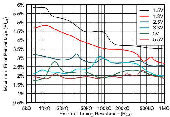
图 5-25. C_{ext} = 1\text{nF} 时最大输出脉冲宽度误差 (绝对值) 与时序电阻器值间的关系
