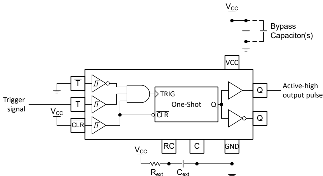
图 8-1. 使用 TPUL2G122x 的脉冲发生器原理图
