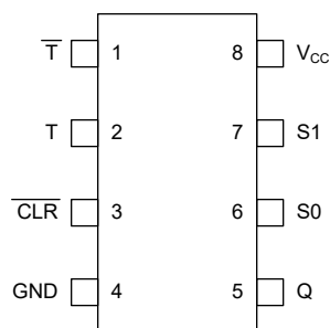
图 4-1. TPUL1G513-Q1 DRL 封装 ( 顶视图 )
