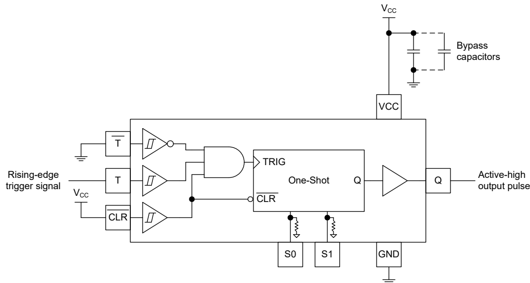
图 8-1. 使用 TPUL1G513-Q1 的脉冲发生器原理图
