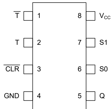
引脚排列图
