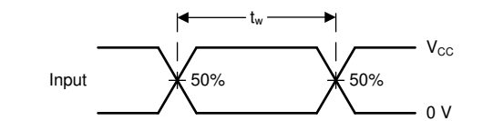
图 6-2. 电压波形，脉冲持续时间
