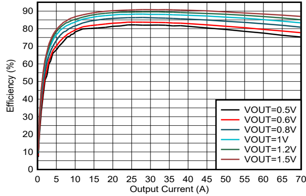
图 5-1. TPSM8D6C24 效率与输出电流间的关系
