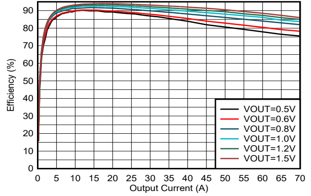
图 5-2. TPSM8D6C24 效率与输出电流间的关系
