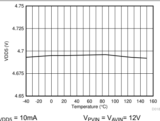
图 5-12. VDD5 电压与结温间的关系
