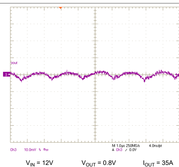
图 8-8. V_{OUT} 稳态纹波
