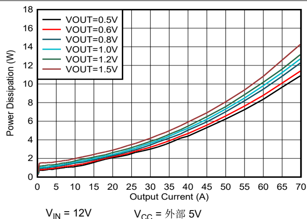
图 5-8. TPSM8D6C24 功率耗散与输出电流间的关系
