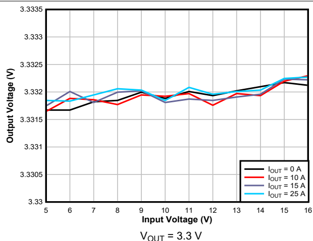
图 8-6. Line Regulation
