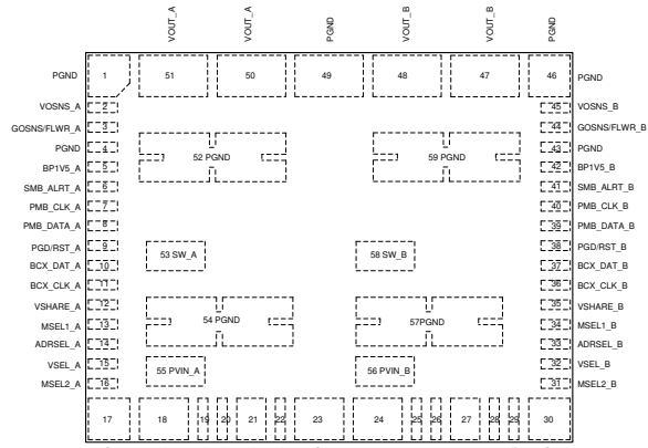
图 5-1. 59-Pin QFM-MOW Package (Top View)
