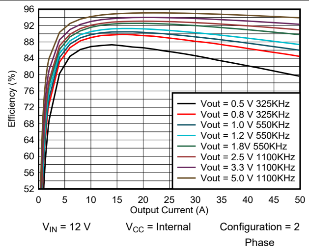
图 6-4. TPSM8D6B24 Efficiency vs Output Current
