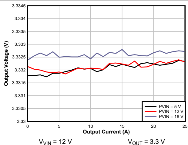
图 8-4. Load Regulation
