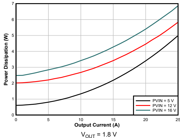
图 8-7. Power Dissipation
