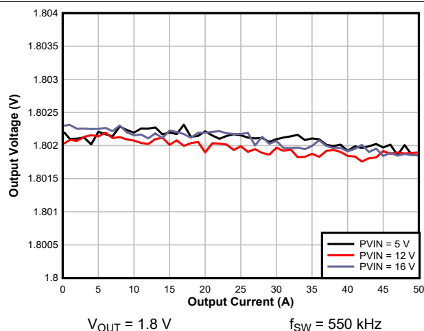
图 8-19. Load Regulation
