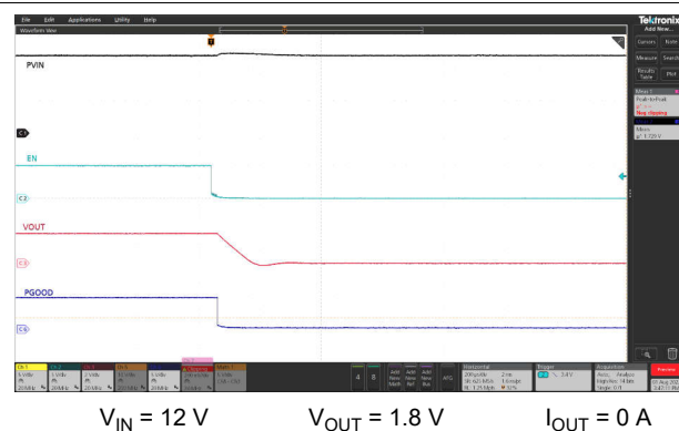
图 8-11. Enable Shutdown
