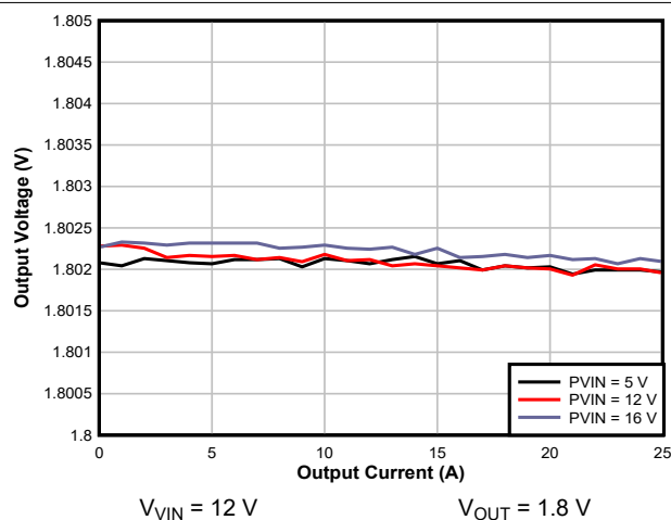
图 8-3. Load Regulation
