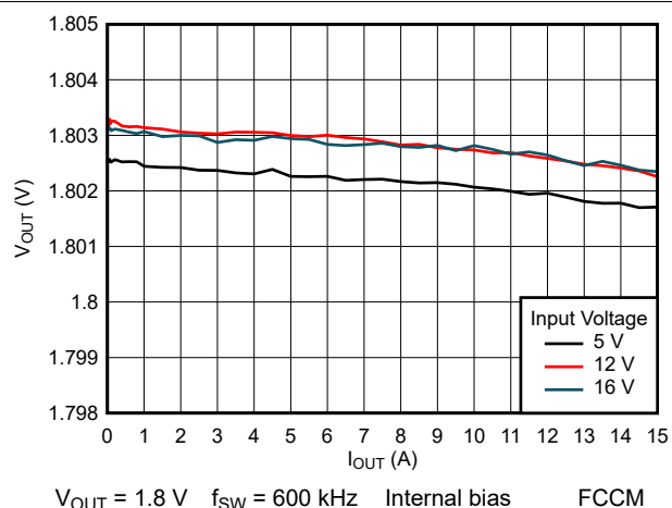
图 8-15. Load Regulation
