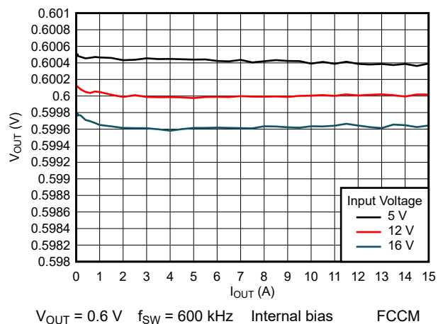
图 8-11. Load Regulation
