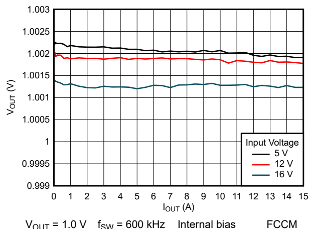
图 8-13. Load Regulation
