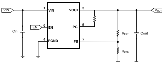
简化原理图
