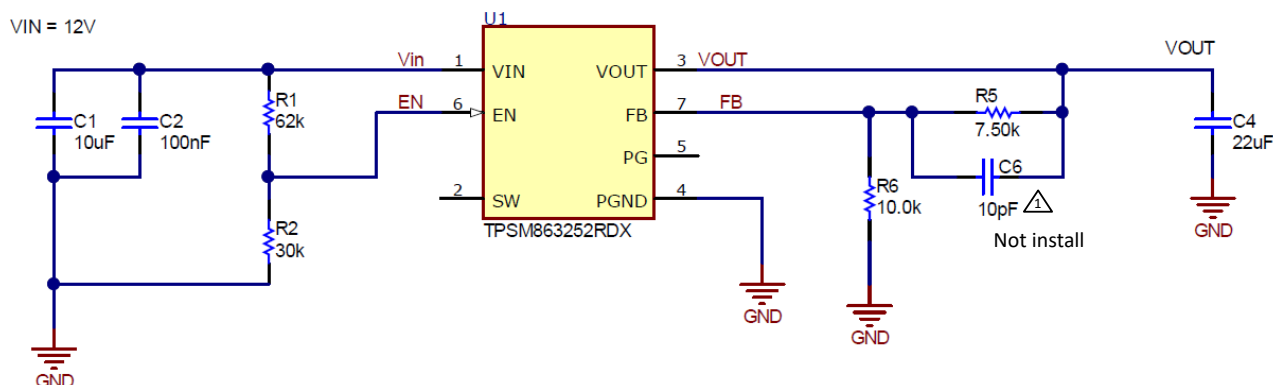
图 8-1. Schematic
