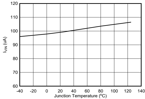
图 6-1. TPSM863252 Quiescent Current
