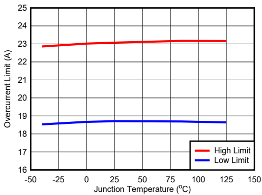
图 6-3. 过流限值
