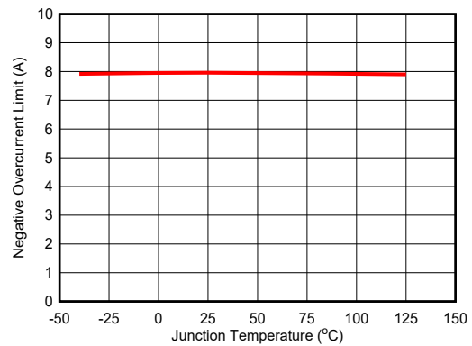
图 6-4. 负过流限制
