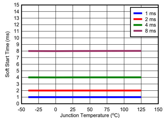
图 6-12. 软启动
