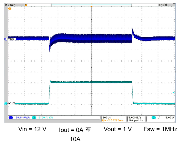
图 8-8. 负载瞬态
