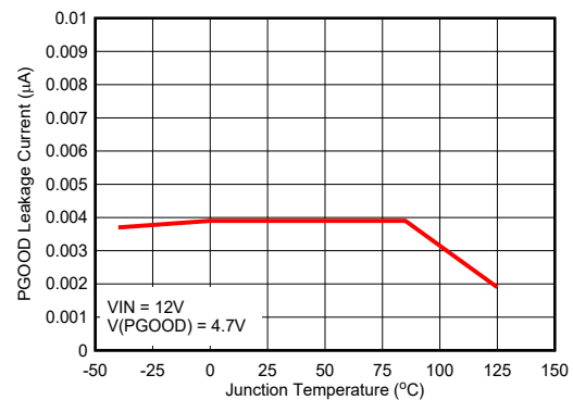
图 6-10. PG 漏电流
