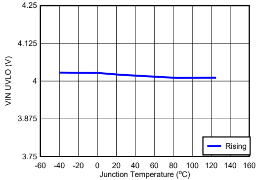
图 6-7. VIN UVLO
