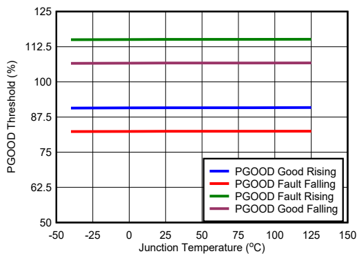
图 6-9. PG 阈值
