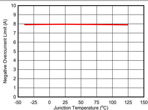
图 6-4. 负过流限制
